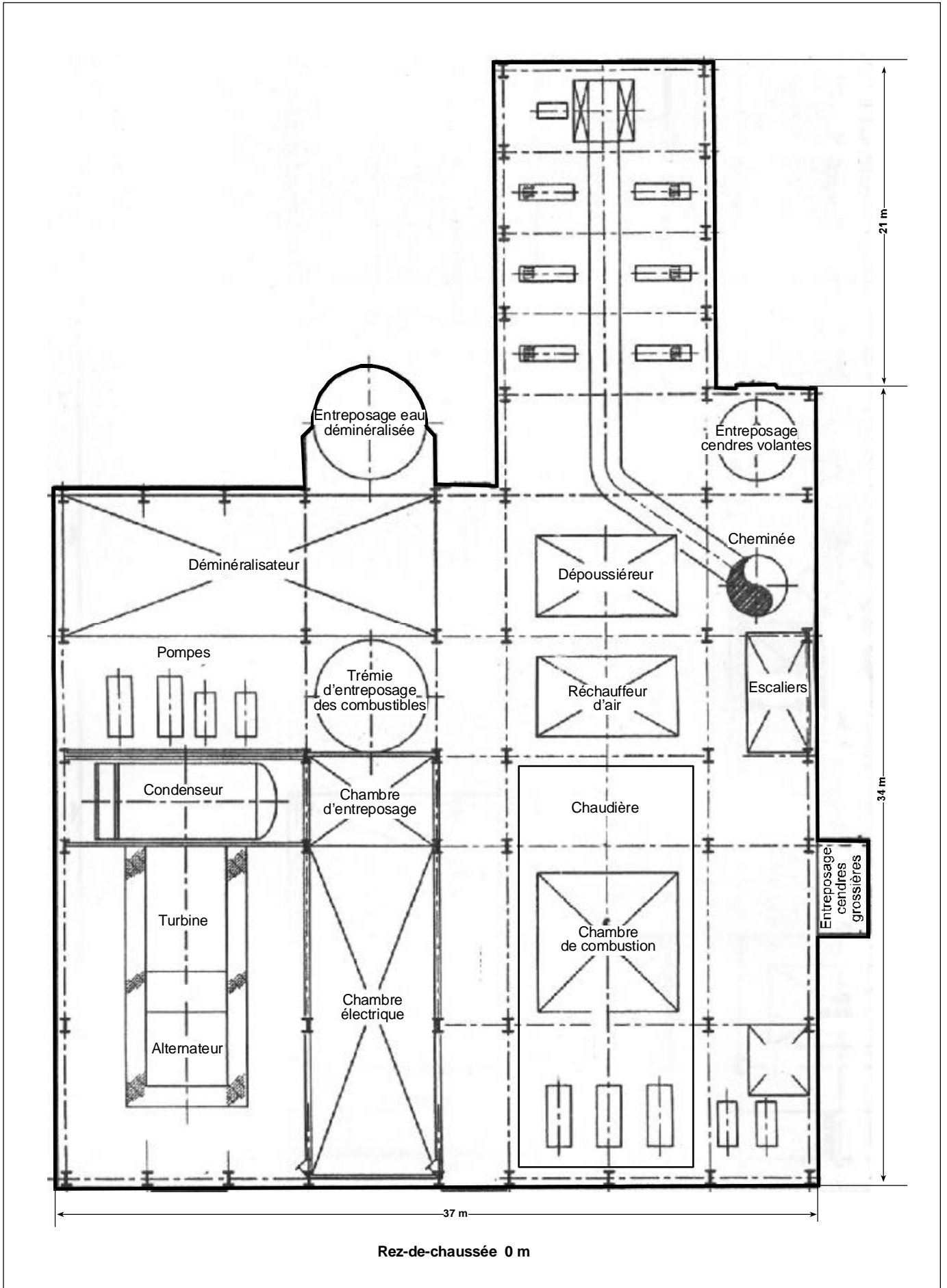
Figure 11. Exemple d'un bâtiment abritant une chaudière et un turboalternateur - Vue en plan
