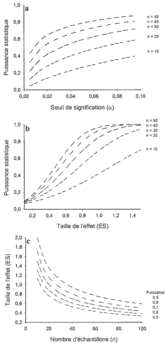
Figure 4 : Variation de différents paramètres statistiques obtenus à partir de données fictives. L'analyse utilisée est un test de t pour échantillons indépendants. (a) Variation de la puissance statistique selon le seuil de signification pour différentes tailles d'échantillons ( n ). (b) Variation de la puissance statistique selon la taille de l'effet pour différentes tailles d'échantillons. (c) Taille de l'effet nécessaire selon le nombre d'échantillons pour obtenir différentes puissances statistiques.
