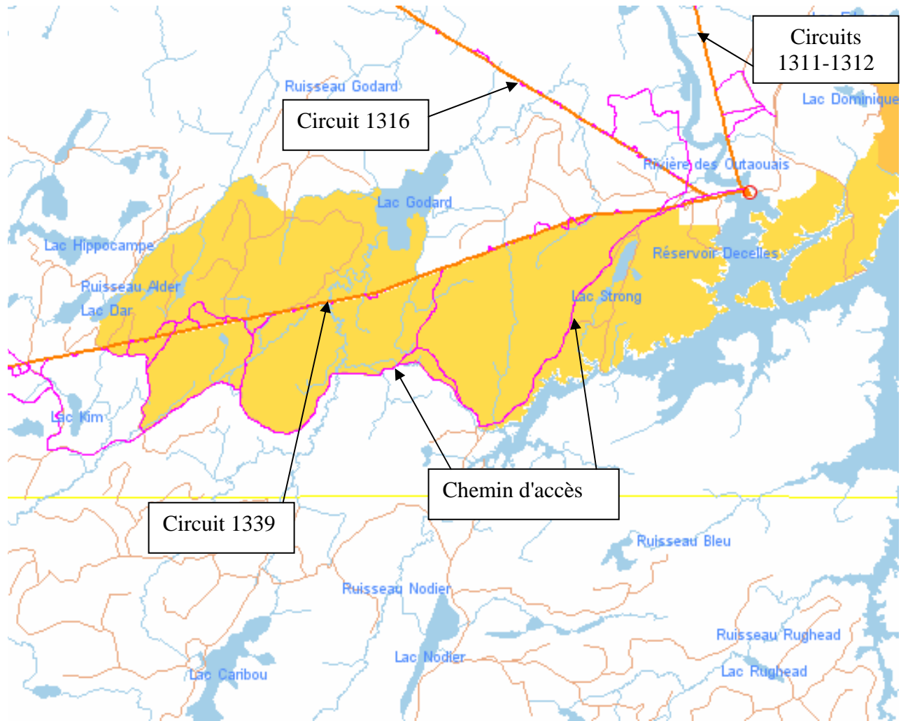
Figure 15 : Circuit 1339 et chemins d'accès RBP Réservoir Decelles
