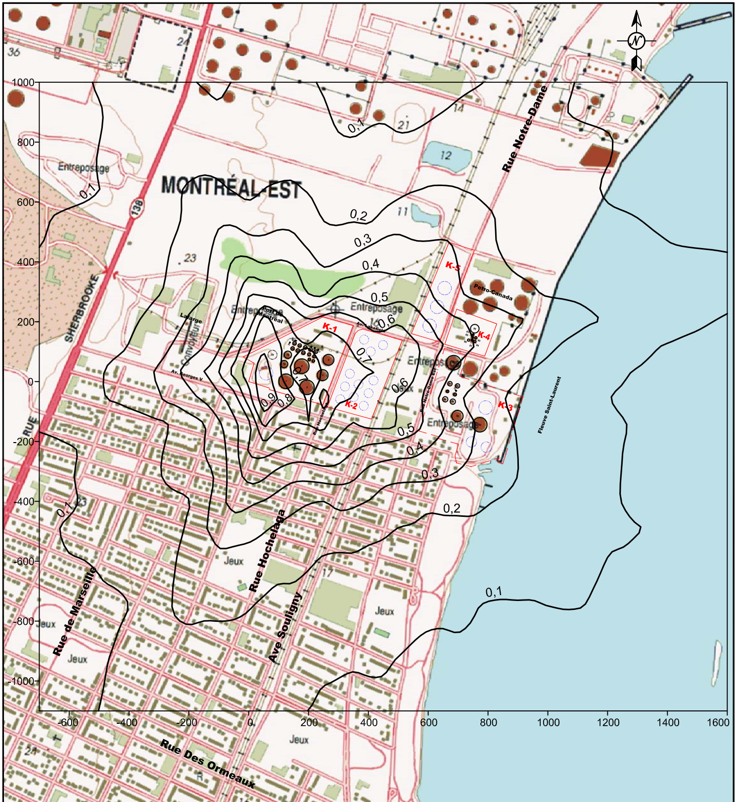
FIGURE 4-2 DISTRIBUTION GÉOGRAPHIQUE DES CONCENTRATIONS MOYENNES JOURNALIÈRES AU NIVEAU DU SOL POUR LE BENZÈNE DANS L'AIR AMBIANT (en ng/m³) SITUATION FUTURE
