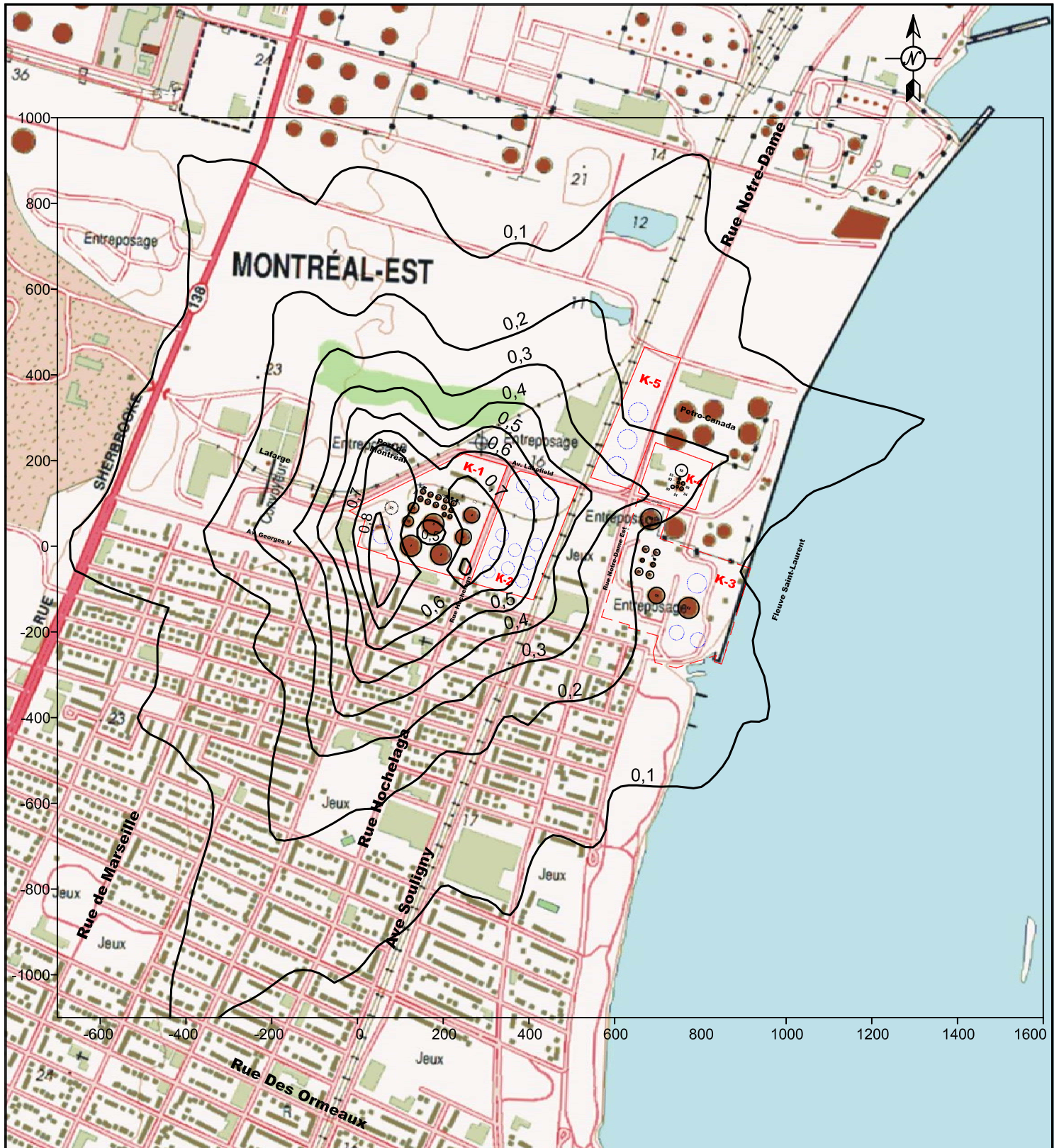
FIGURE 4-1 DISTRIBUTION GÉOGRAPHIQUE DES CONCENTRATIONS MOYENNES JOURNALIÈRES AU NIVEAU DU SOL POUR LE BENZÈNE DANS L'AIR AMBIANT (en ng/m 3 ) SITUATION ACTUELLE
