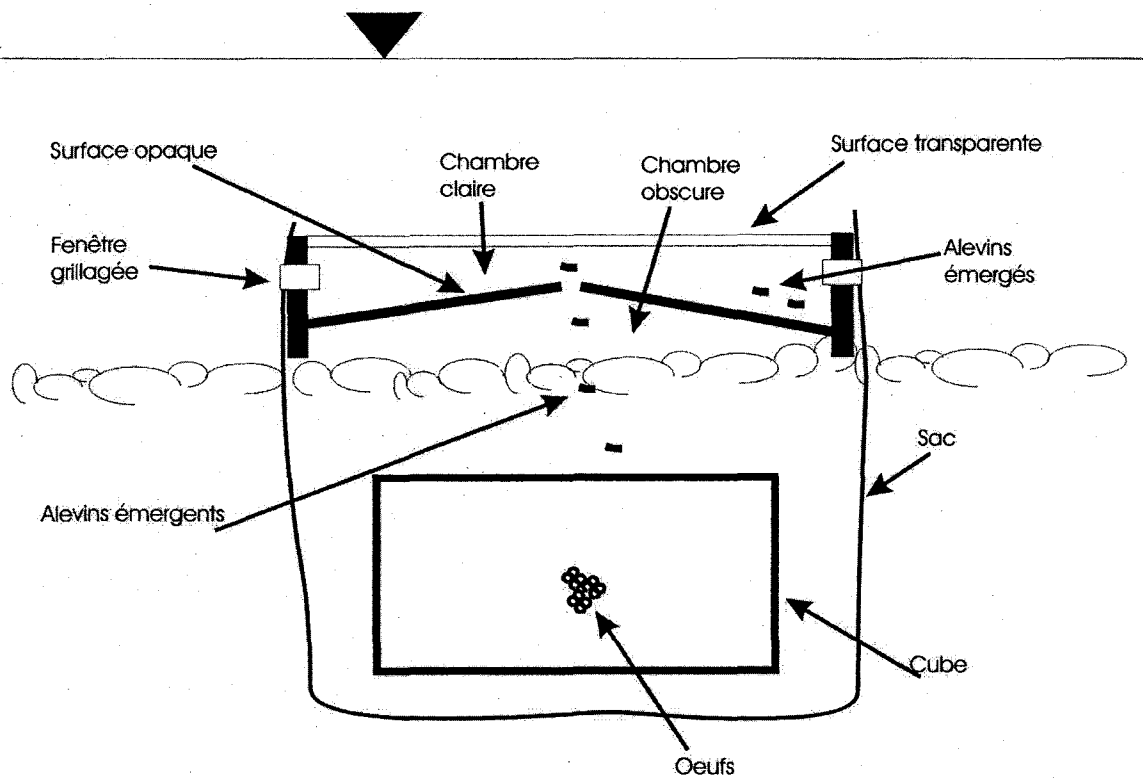
Figure 9. Schéma d'un panier muni d'une trappe d'émergence.
