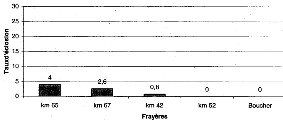
Figure 23. Taux d'éclosion des œufs sur les différentes frayères au 28 juin 2004..
