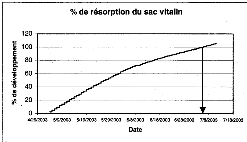
Figure 20. Évolution estimée du pourcentage de résorption du sac vitellin des alevins.
