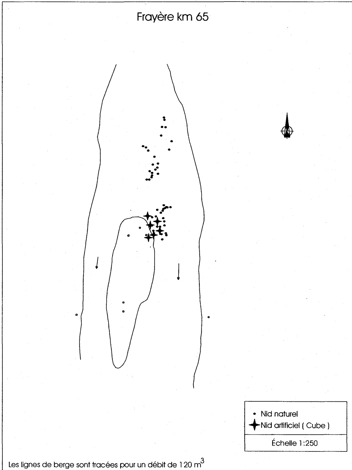
Figure 3. Carte de la frayère du kilomètre 65.
