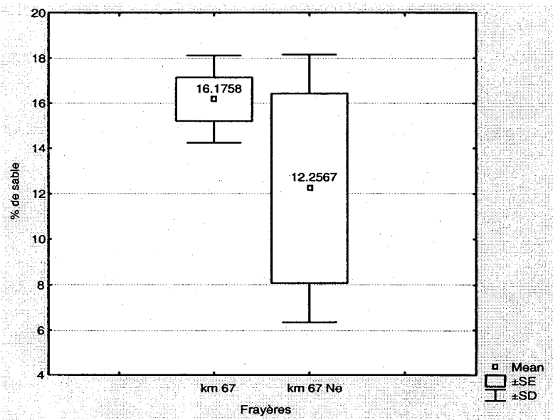
Figure 29. Pourcentage de sables et silts (< 2 mm) mesuré au printemps dans les paniers d'incubation sur les zones nettoyées et non-nettoyées à l'automne.
