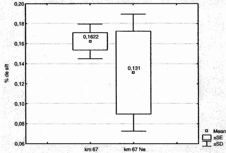
Figure 30. Pourcentage de silt (< 0.063 mm) mesuré au printemps dans les paniers d'incubation sur les zones nettoyées et non-nettoyées à l'automne.
