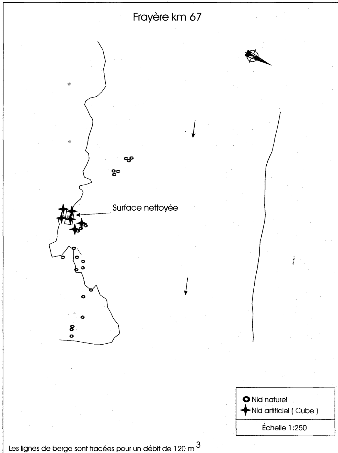
Figure 2. Carte de la frayère du kilomètre 67.
