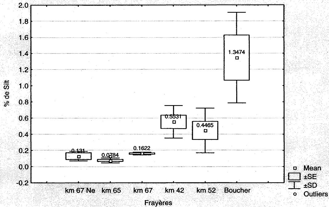
Figure 25. Pourcentage de silts (< 0.063 mm) mesuré dans les paniers d'incubation des différentes frayères.
