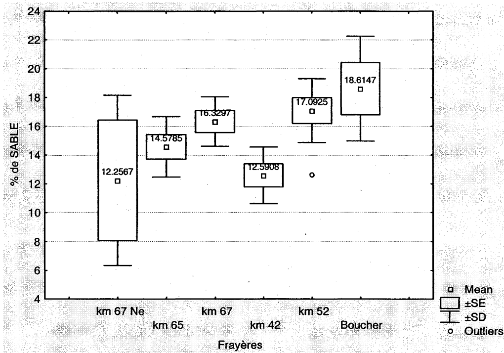
Figure 26. Pourcentage de sables et silts (< 2 mm) mesuré dans les paniers d'incubation des différentes frayères.
