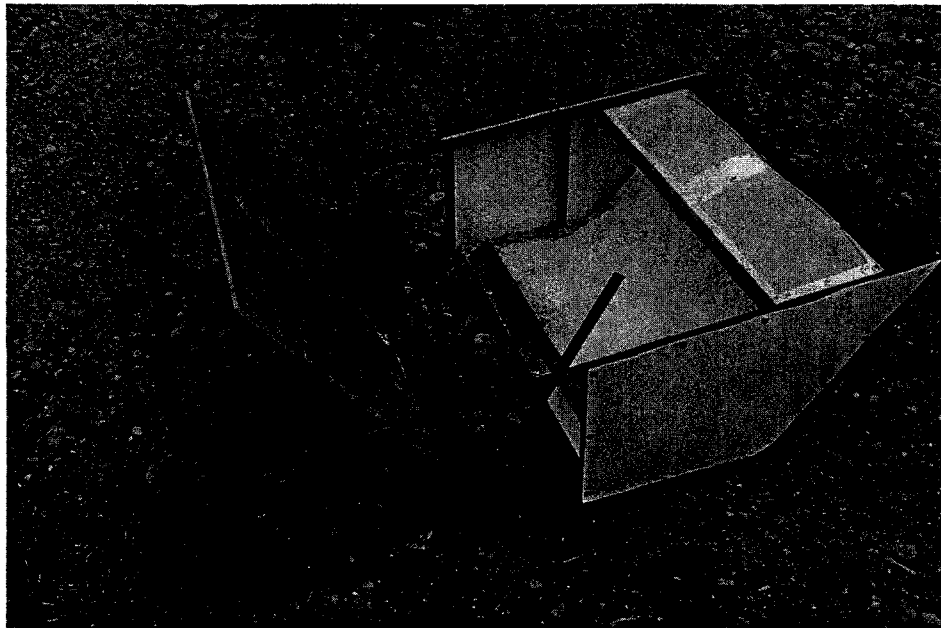
Figure 14. Photo du traîneau déflecteur adapté à la récupération des sédiments.
