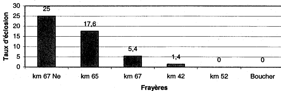
Figure 22. Taux d'éclosion des œufs sur les différentes frayères au 7 juin 2004.
