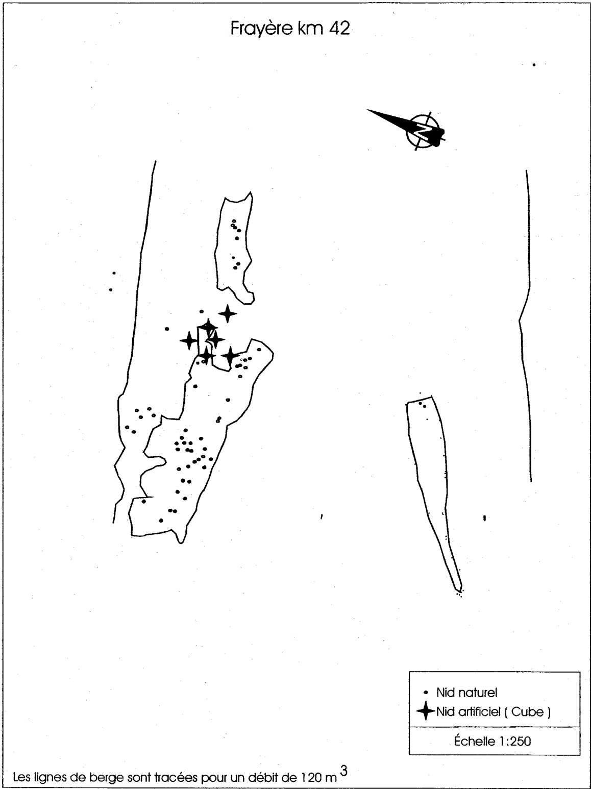
Figure 5. Carte de la frayère du kilomètre 42.
