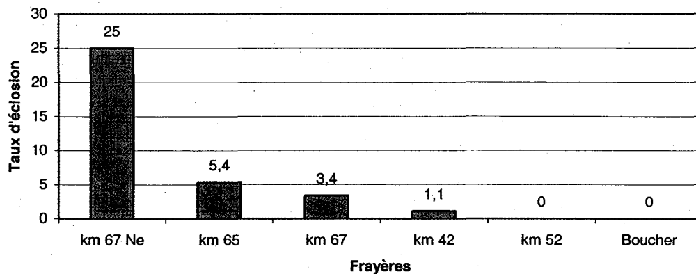
Figure 24. Taux d'éclosion des oeufs sur les différentes frayères en combinant ensemble les relevés du 7 et 28 juin.
