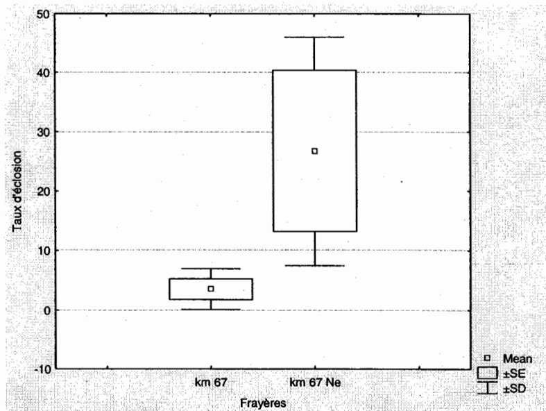
Figure 31. Comparaison des taux d'éclosion des oeufs entre les zones nettoyées et non-nettoyées sur la frayère km 67.
