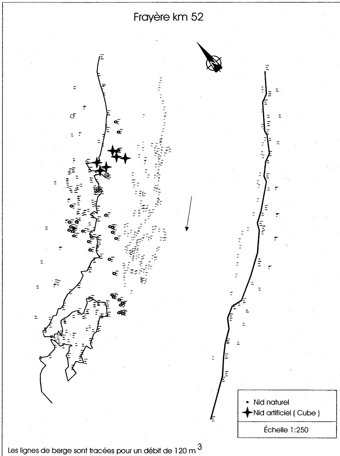
Figure 4. Carte de la frayère du kilomètre 52.
