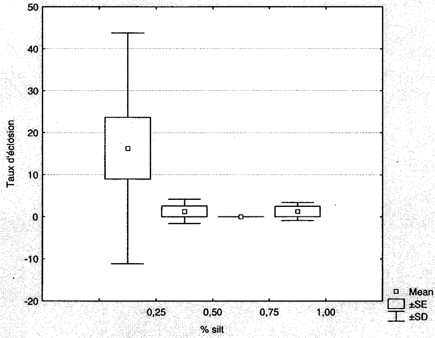
Figure 27. Relation entre le taux d'éclosion des œufs et le pourcentage de silts (<0.063mm).
