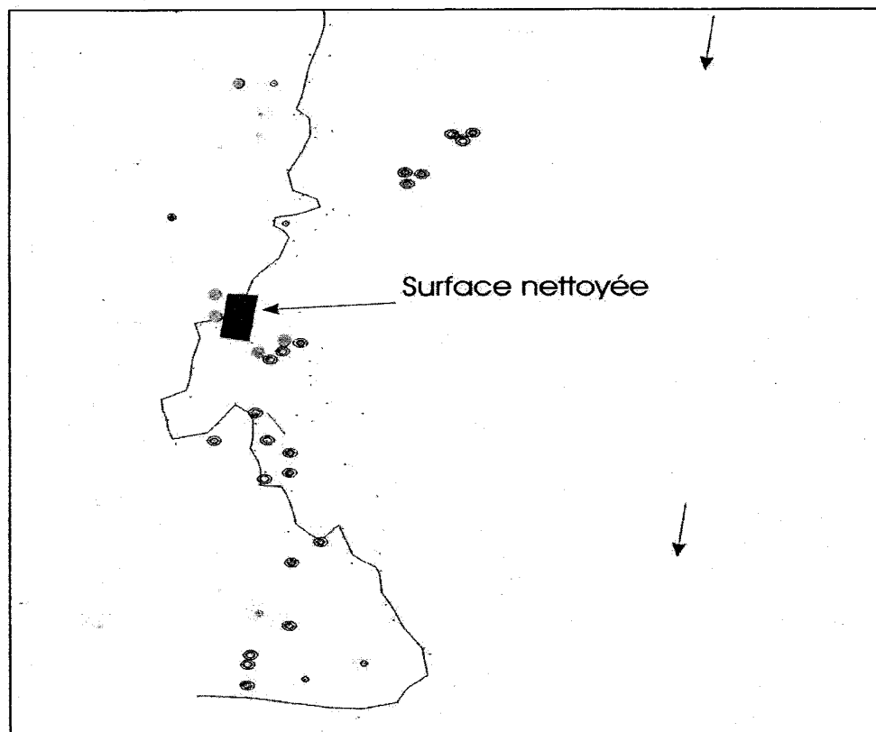
Figure 13. Carte de la surface nettoyée sur la frayère km 67.
