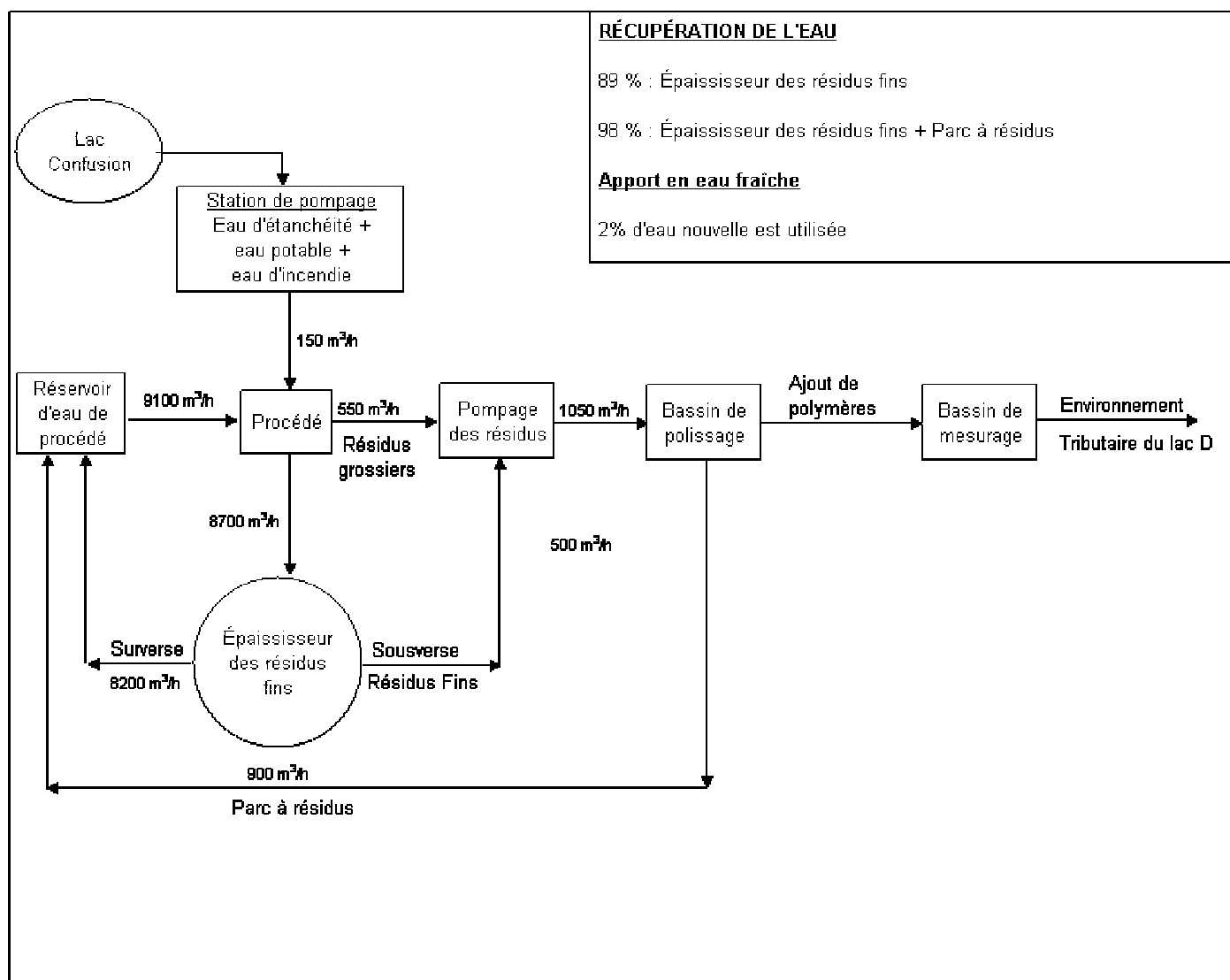
Figure 3.6 Bilan de l'eau global en condition normale d'opération
