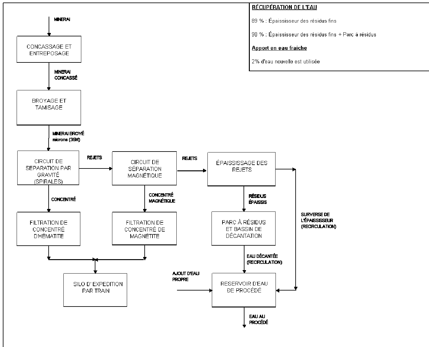
Figure 3.5 Diagramme du processus de traitement du minerai
