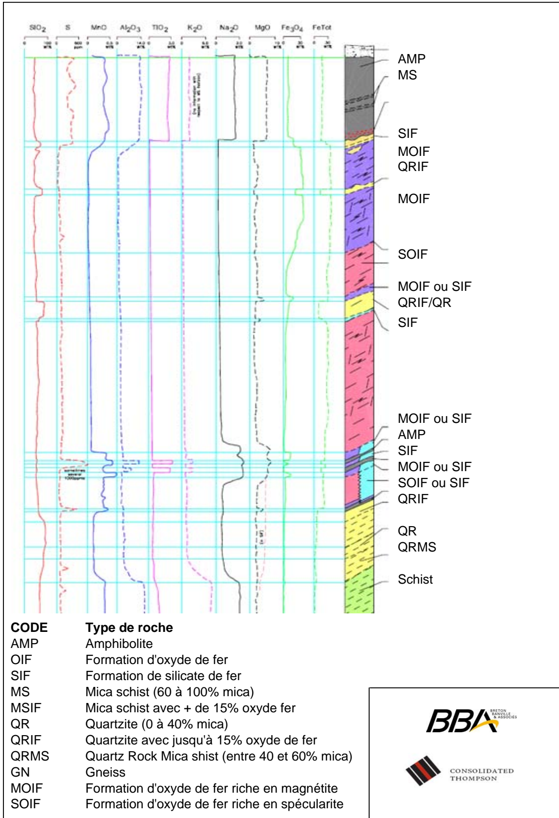
Figure 3.2 Section typique du dépôt du lac Bloom
