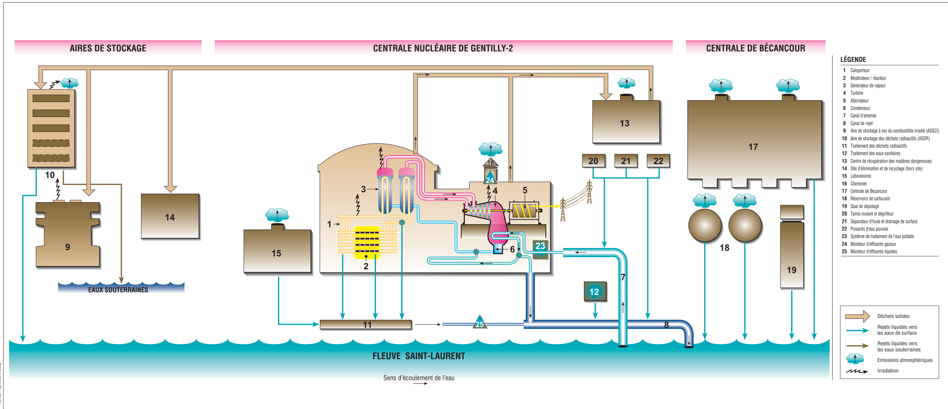
Figure 3-1 : Schéma simplifié des principales sources de rejets
