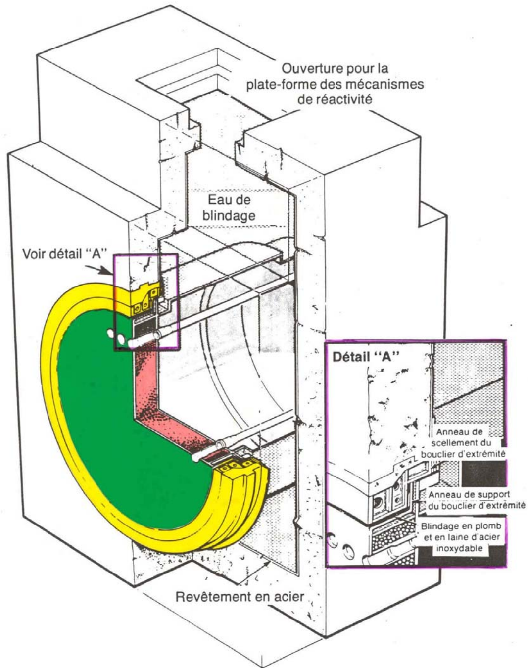
Caisson en béton du réacteur
