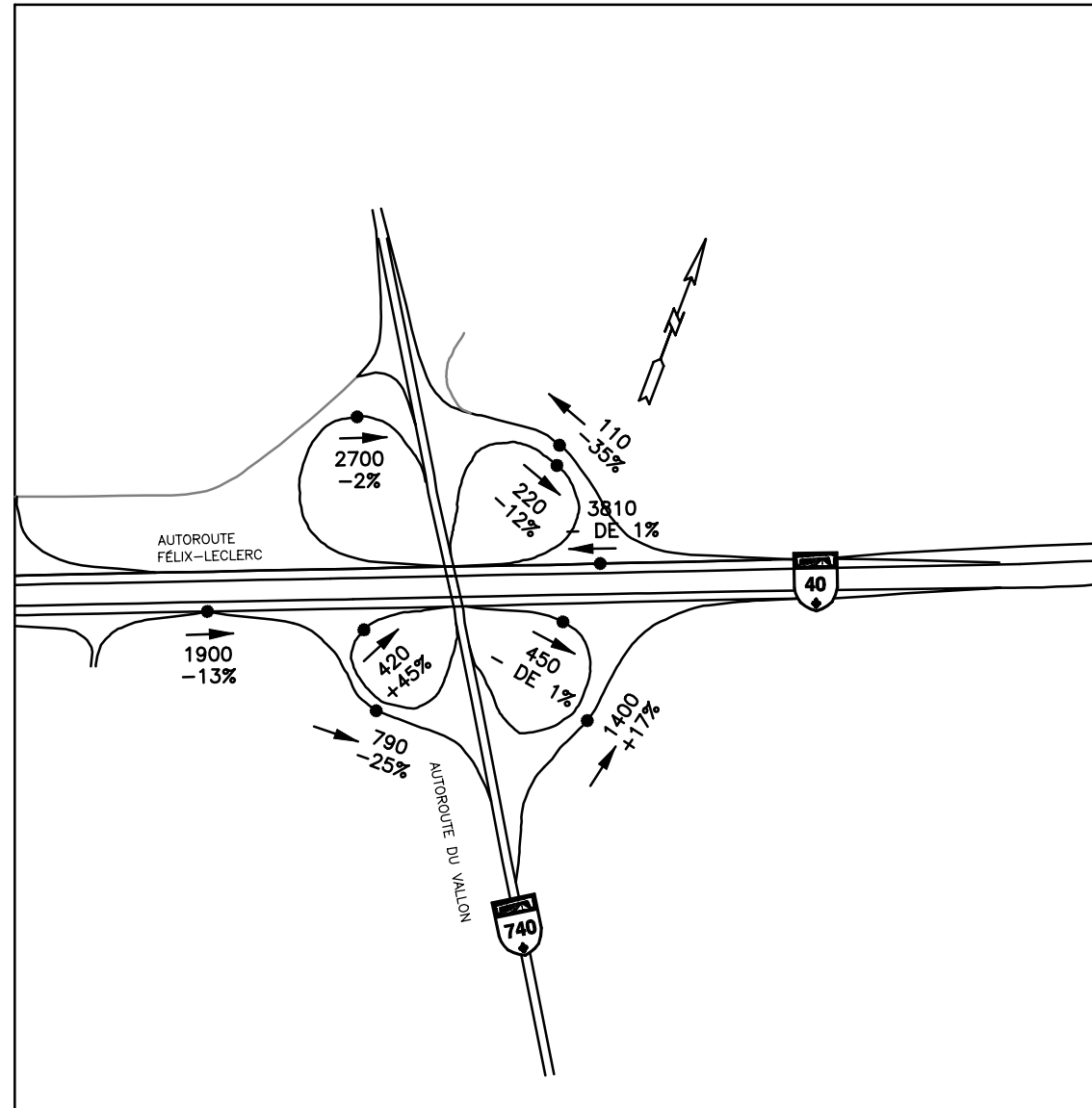
AGRANDISSEMENT ÉCHANGEUR AUTOROUTES DU VALLON (740) ET FÉLIX-LECLERC (40)
