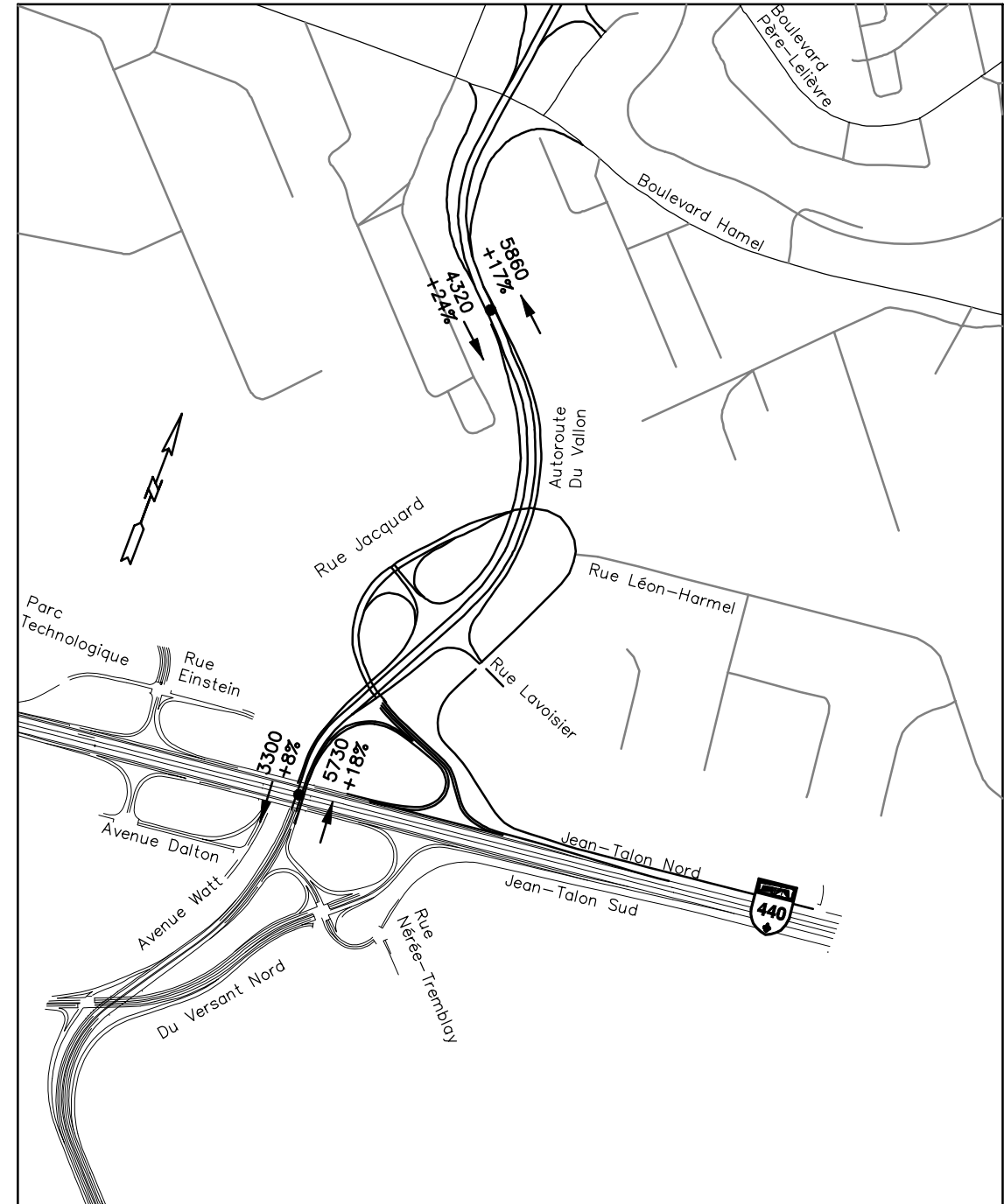
AGRANDISSEMENT ÉCHANGEUR AUTOROUTES DU VALLON (740) ET CHAREST (440)
