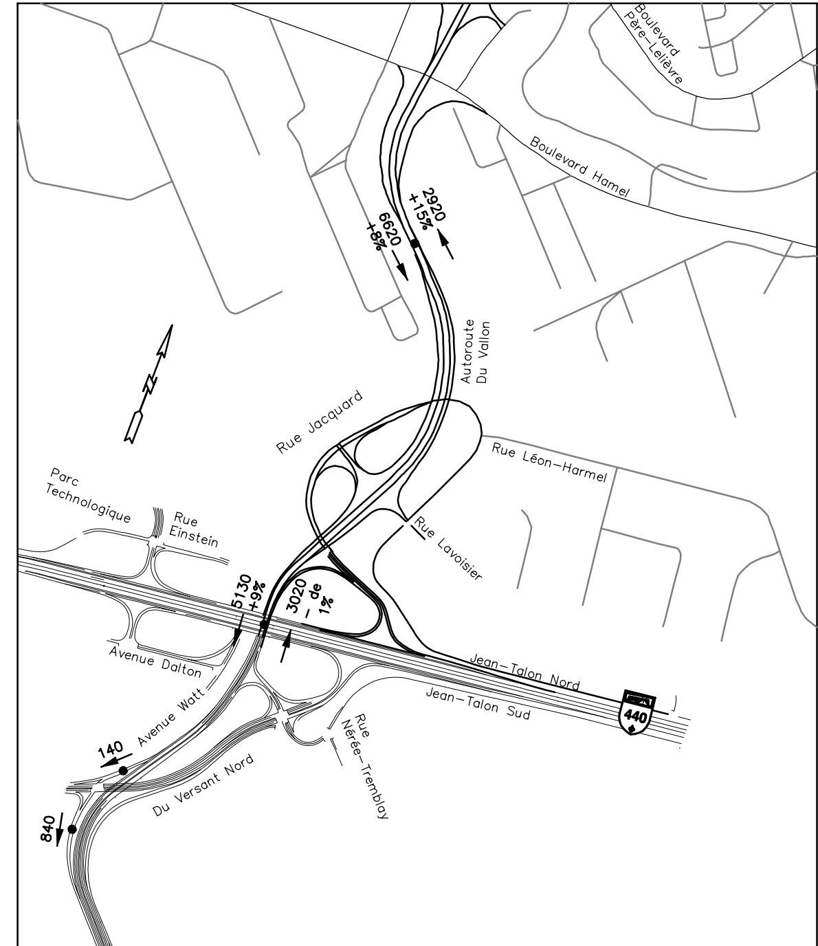
AGRANDISSEMENT ÉCHANGEUR AUTOROUTES DU VALLON (740) ET CHAREST (440)
