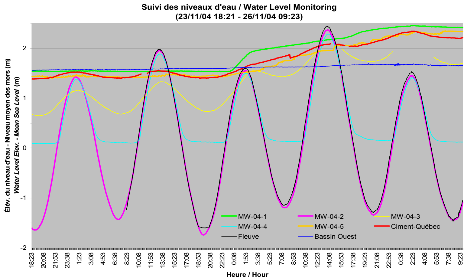
Figure 4 Suivi piézométrique (23 au 26 novembre 2004)
