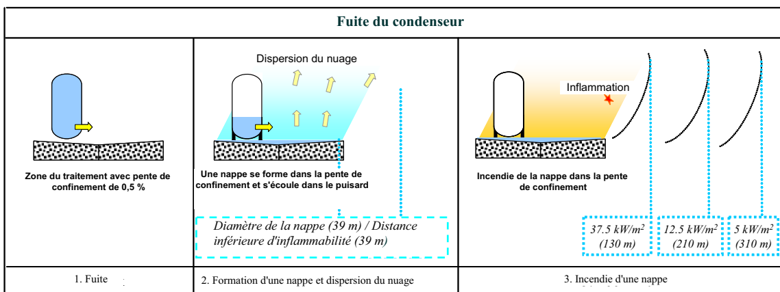
Figure 9.4-5 Illustration d'une fuite de condenseur
