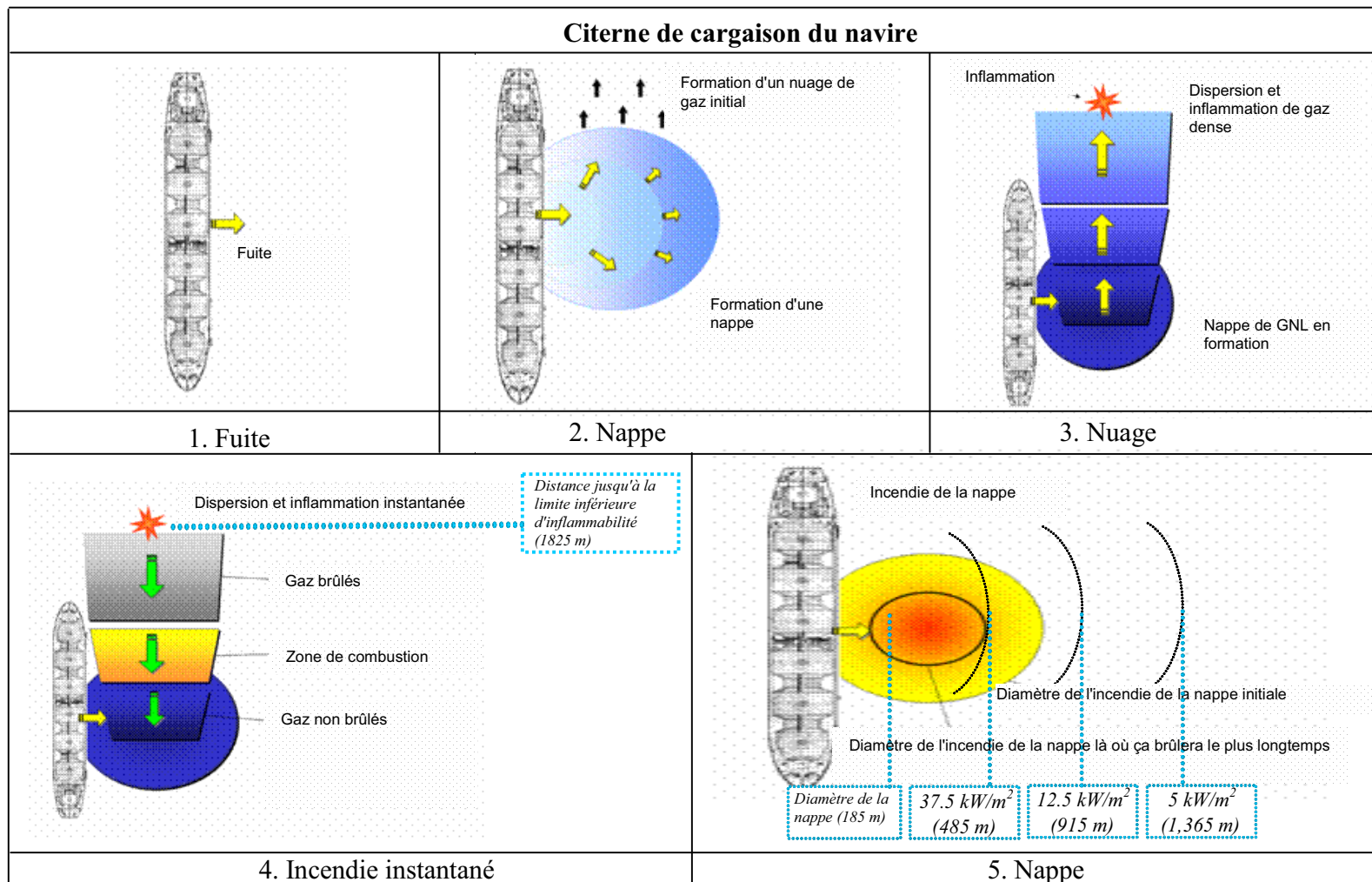
Figure 9.4-2 Illustration d'une fuite d'un réservoir de méthancier
