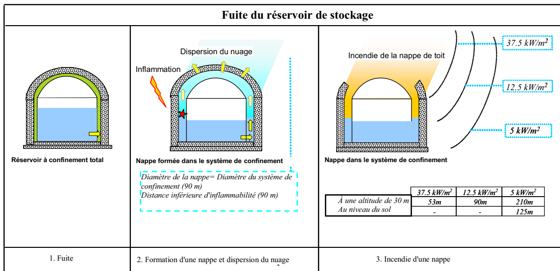
Figure 9.4-4 Fuite du réservoir de stockage
