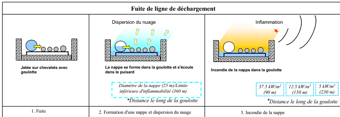
Figure 9.4-3 Illustration d'une fuite de ligne de déchargement
