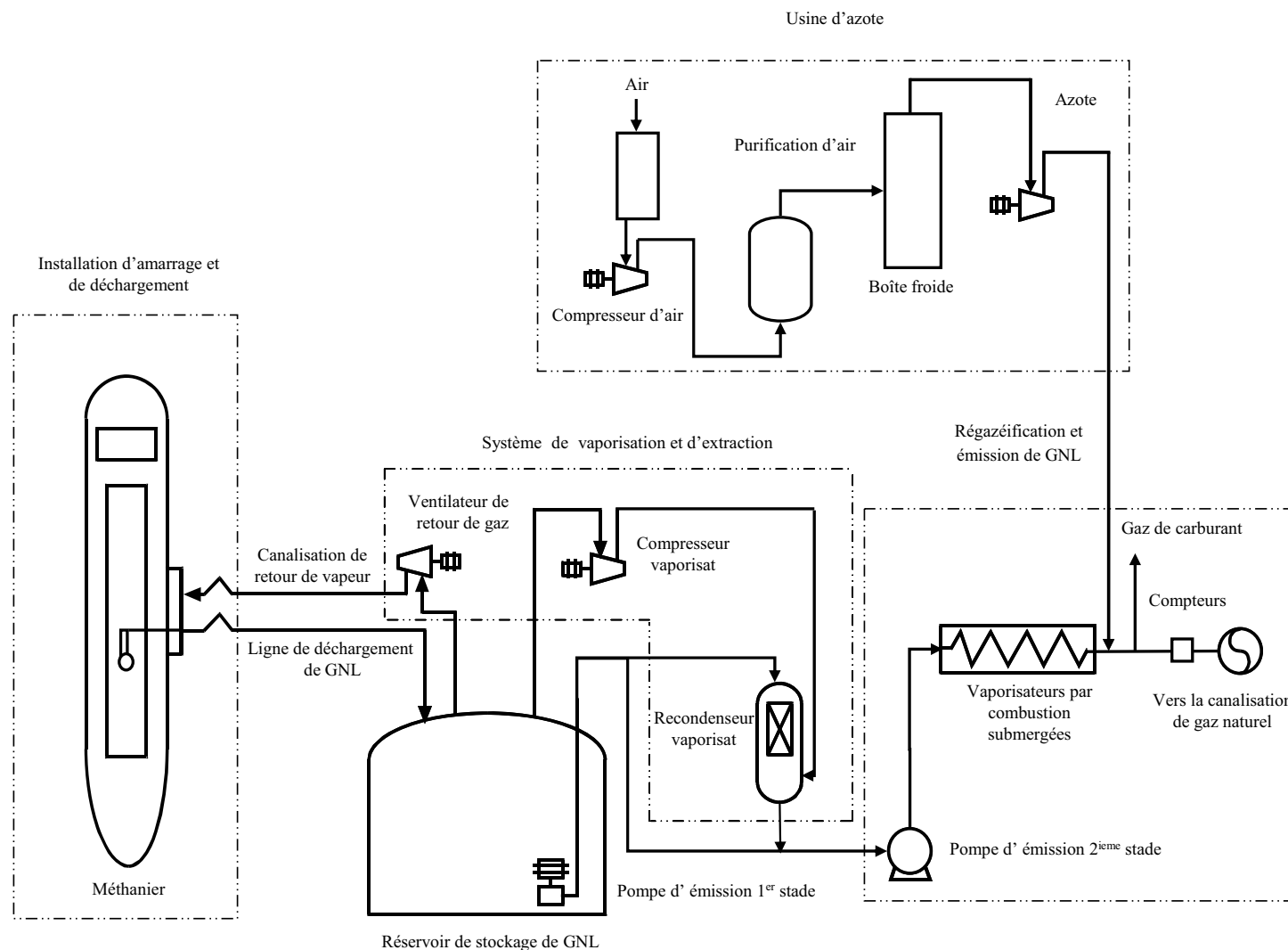
Figure 2.4-6 Schéma du procédé du terminal
