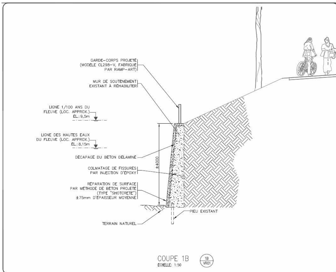
Figure 4. Vue en coupe des travaux de réfection du mur par décapage au tronçon 1 (Source : Génipur, 2016).
