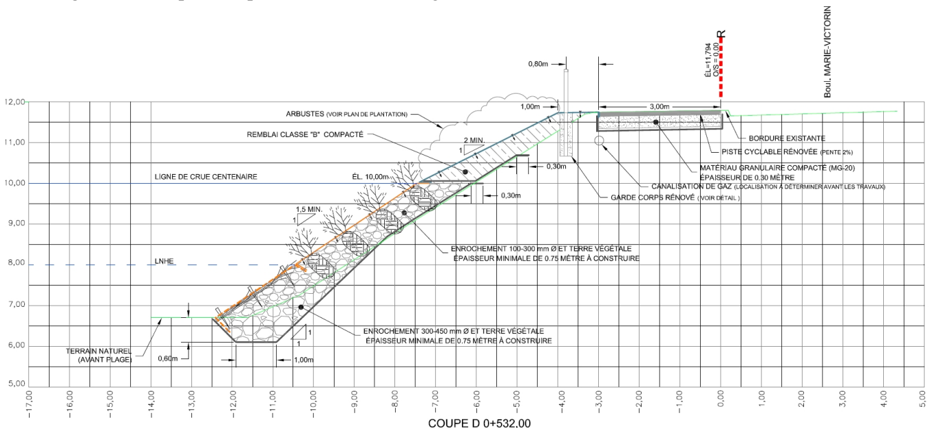
Figure 9. Exemple d'une coupe des travaux de stabilisation de talus en bordure de la piste cyclable «La Riveraine» (Source : Aqua-Berge, 2010).
