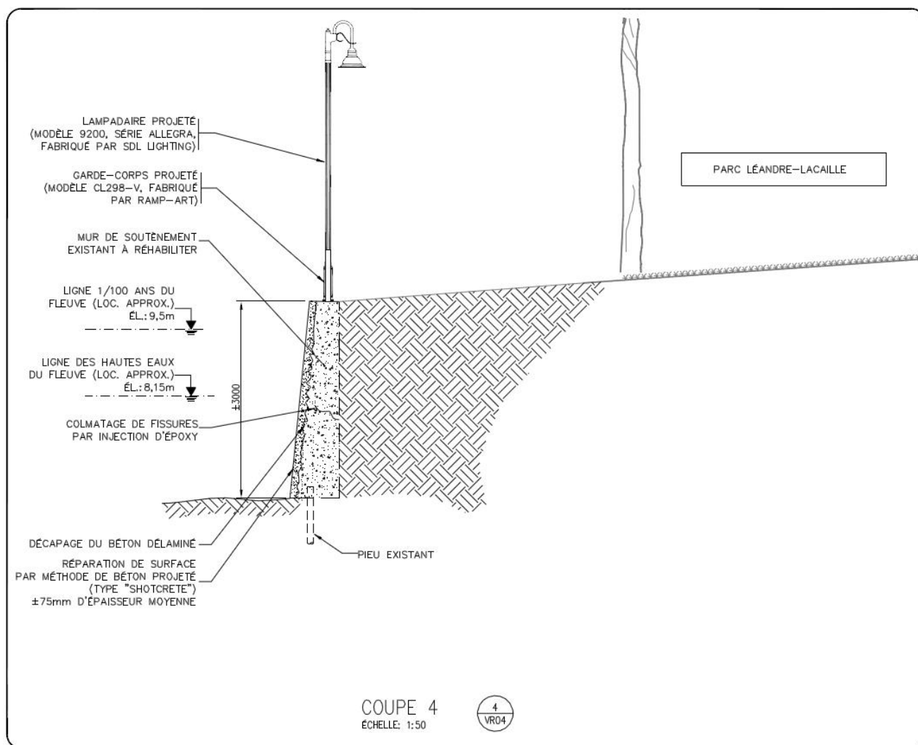
Figure 6. Vue en coupe des travaux de réfection du mur par décapage au tronçon 4 (Source : Génipur, 2015).
