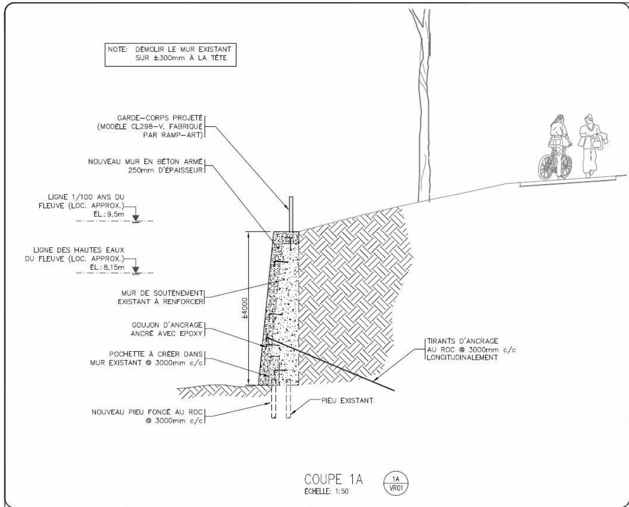
Figure 7. Vue en coupe des travaux de renforcement du mur existant sur les 30 premiers mètres du tronçon 1 (Source : Génipur, 2016)
