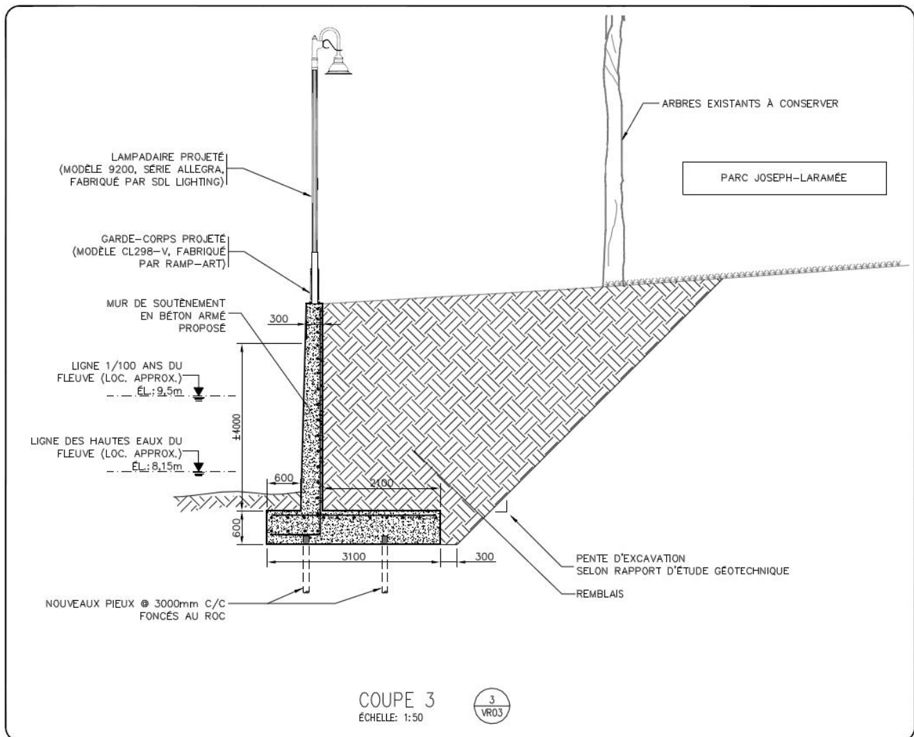
Figure 8. Vue en coupe de la construction d'un nouveau mur de béton au tronçon 3 (Source : Génipur, 2015).
