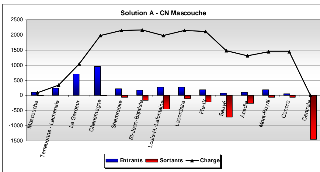
FIGURE 6.3 - Profil de charge de la solution CN - Mascouche - PPAM
