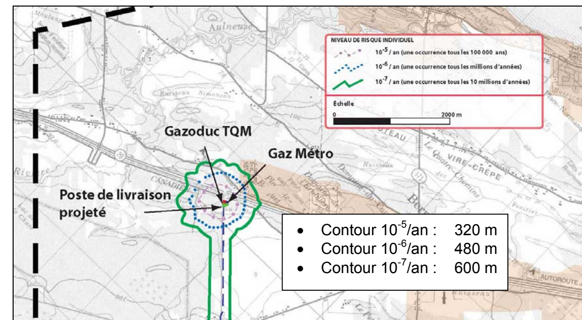
Figure 8.7 Vue élargie des isocontours de risque du gazoduc à la station de raccordement avec le réseau de Gazoduc TQM
