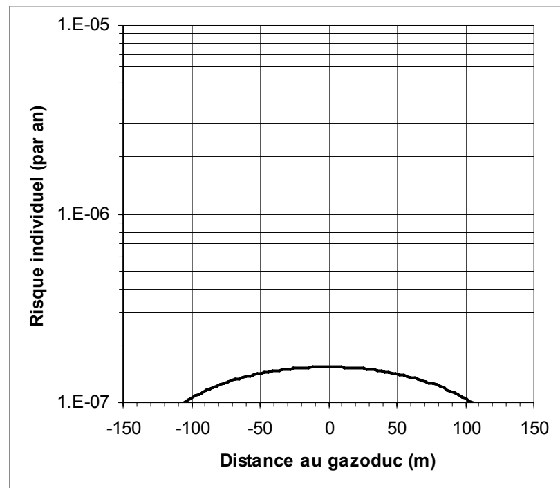
Figure 8.4 Risque individuel en fonction de la distance au gazoduc
