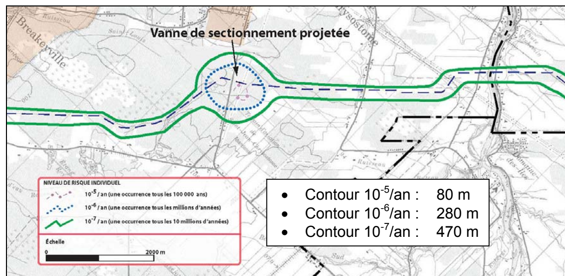
Figure 8.6 Vue élargie des isocontours de risque à la vanne de sectionnement (à mi-chemin)
