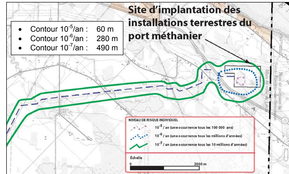
Figure 8.5 Vue élargie des isocontours de risque du gazoduc au point de raccordement au terminal méthanier
