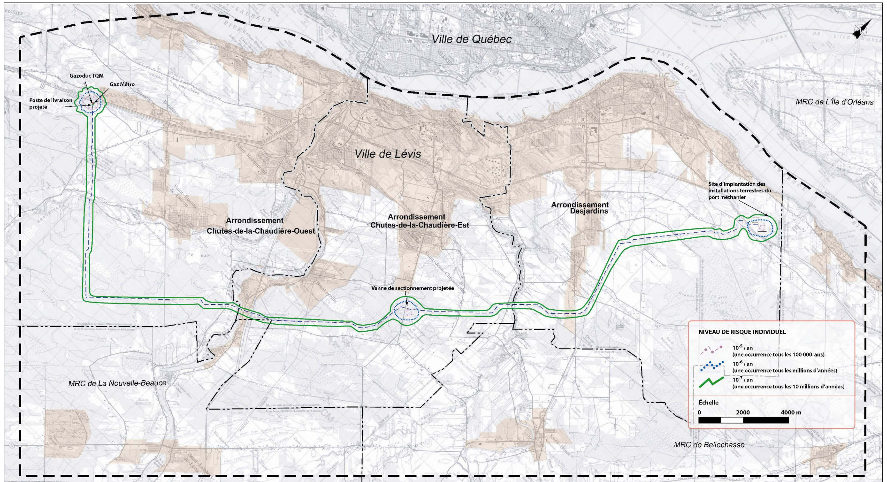
Figure 8.3 Isocontours de risque individuel pour le gazoduc
