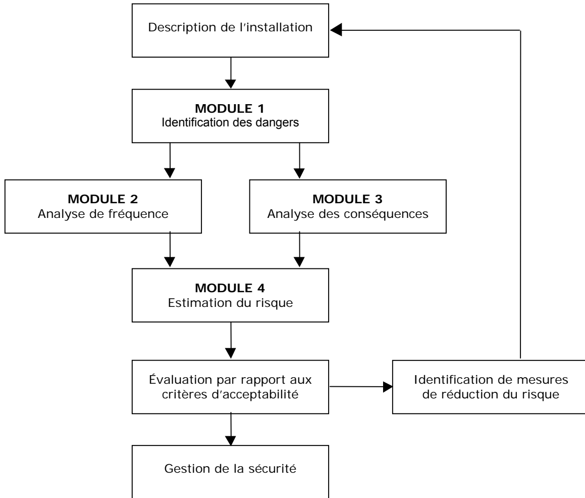
Figure 8.1 Processus d'évaluation du risque et d'itération pour la mise en œuvre des mesures de réduction des risques
