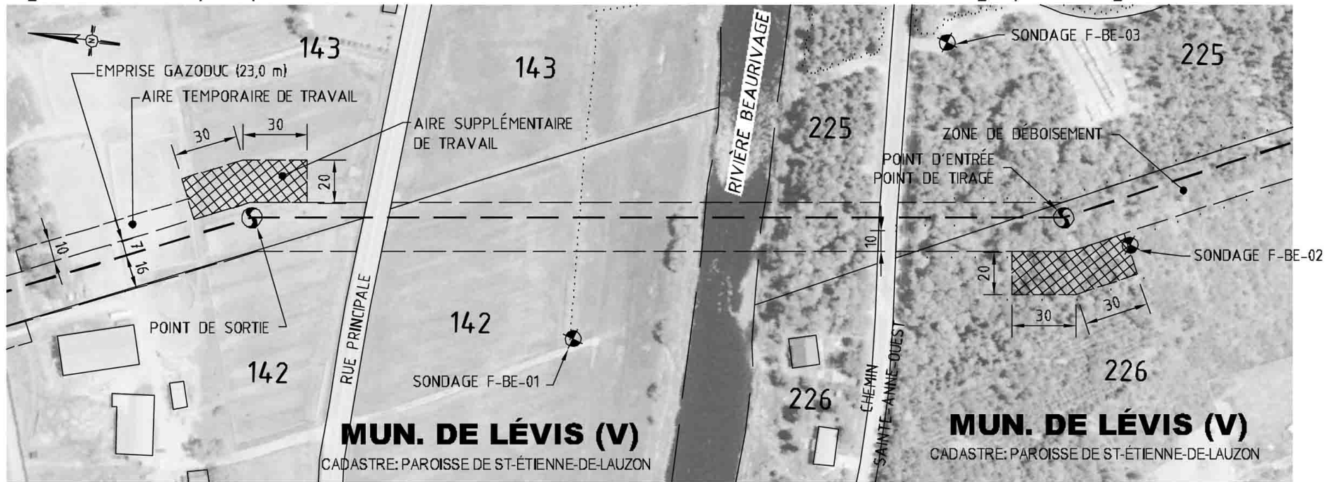
Figure 7.4: Croquis préliminaire associé à la traversée de la rivière Beaurivage par forage directionnel
