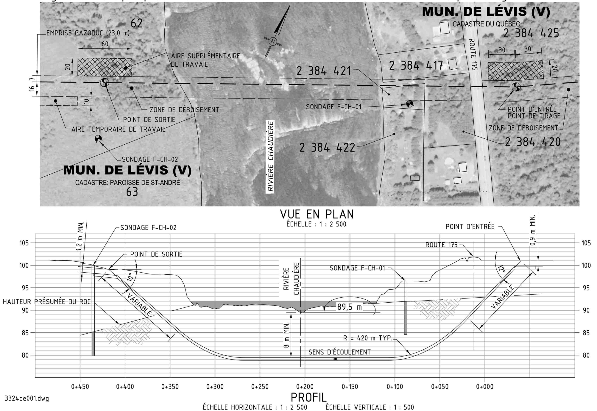
Figure 7.3: Croquis préliminaire associé à la traversée de la rivière Chaudière par forage directionnel
