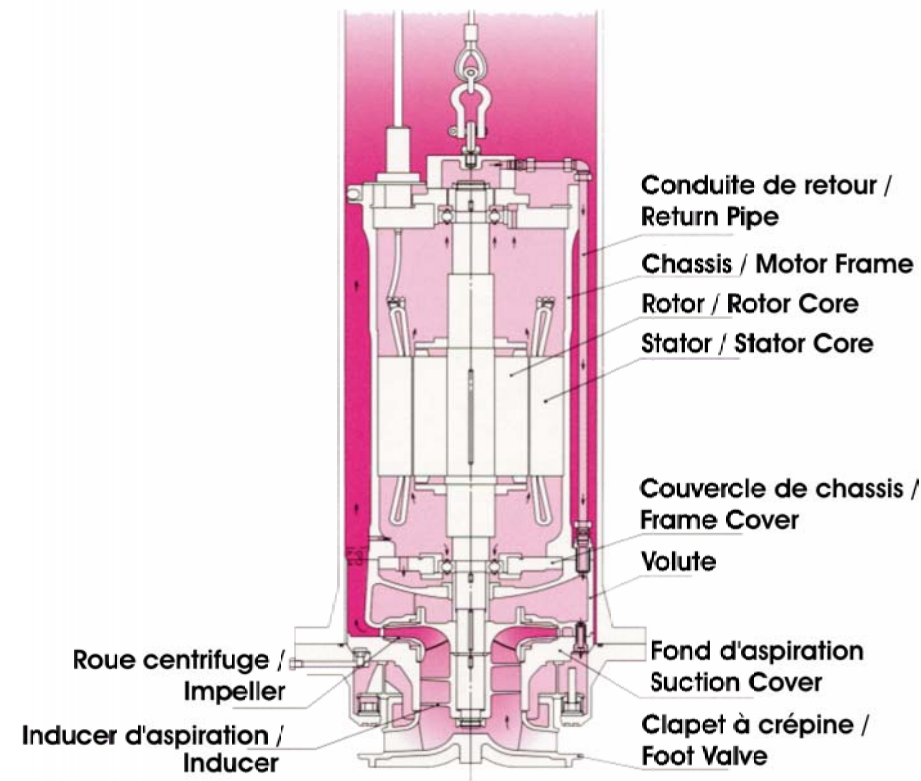
Schéma d'une pompe immergée / Diagram of a Submerged Pump
