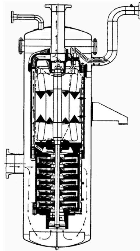
Schéma d'une pompe à barel / Diagram of a Barrel Pump
