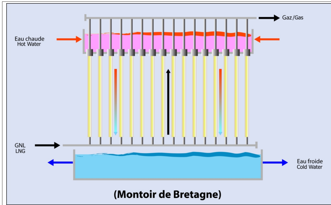
Schéma d'un vaporiseur à ruissellement à eau du terminal méthanier de Montoir-de-Bretagne / Diagram of open rack vaporizer from the Montoir-de-Bretagne LNG terminal
