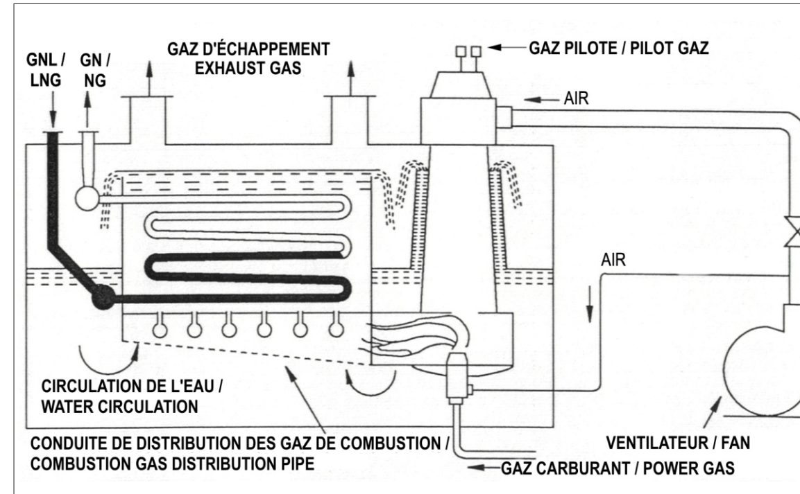
Schéma d'un vaporiseur à combustion submergée du terminal méthanier de Montoir-de-Bretagne / Diagram of the Submerged Combustion Vaporizer from the Montoir-de-Bretagne LNG Terminal
