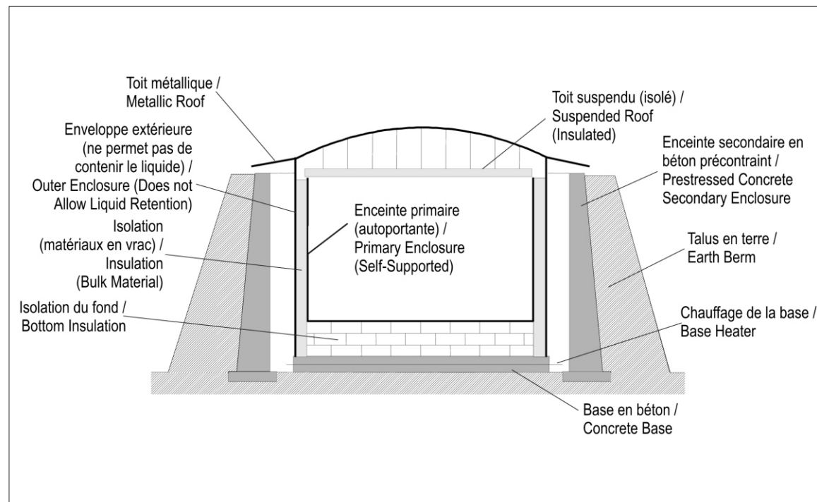
Réservoir à confinement double / Double Containment Tank
