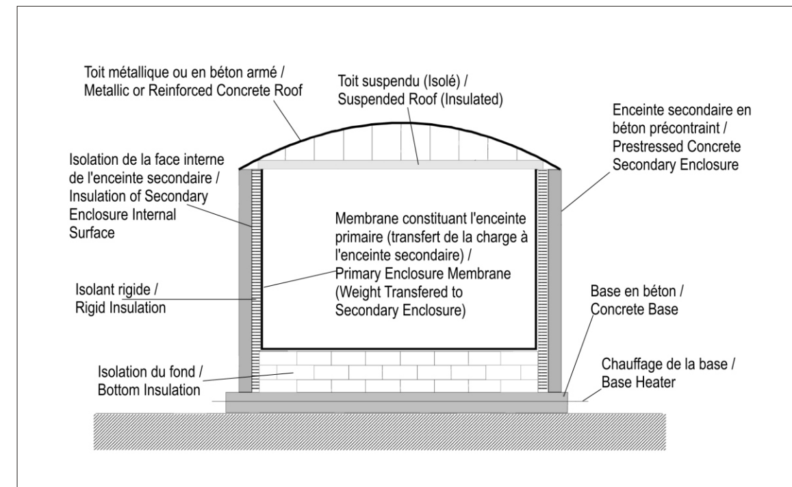
Réservoir à membrane / Membrane Tank
