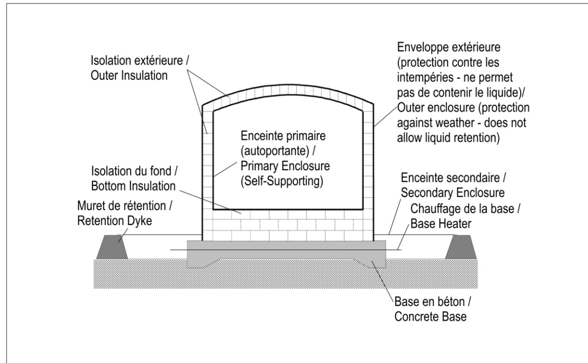
Réservoir à simple intégrité / Single Containment Tank
