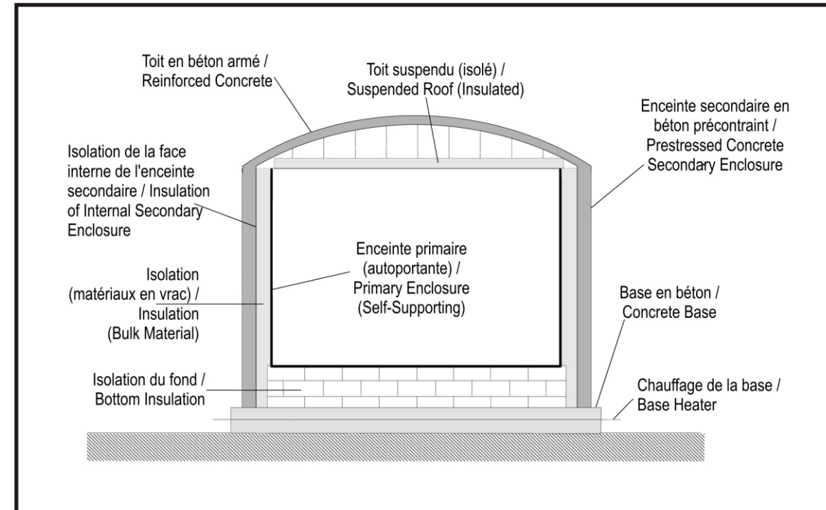
Réservoir à intégrité totale / Full Containment Tank
