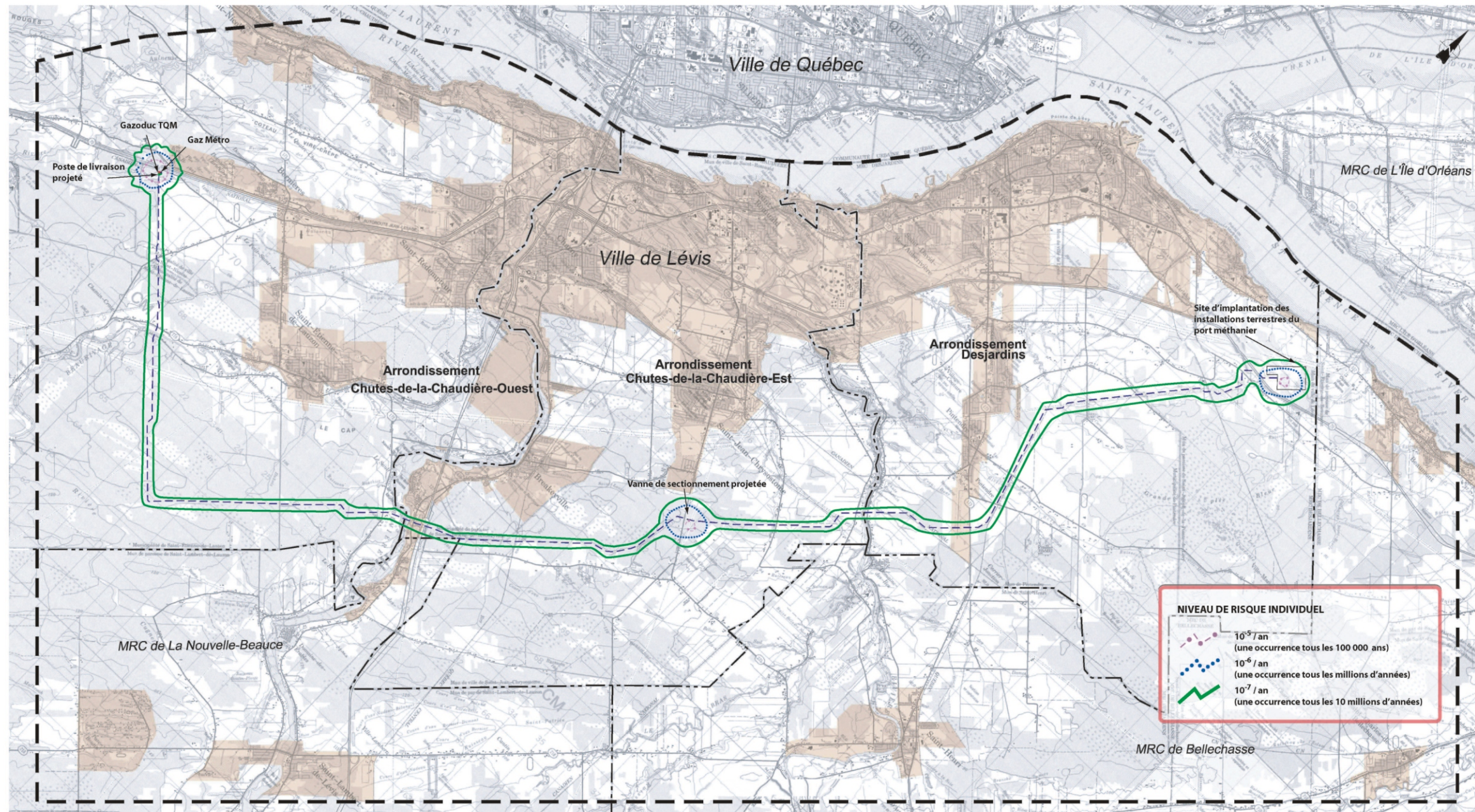
Titre / Title Isocontours de risque individuel pour le gazoduc / Individual Risk Isocontours for the Pipeline
