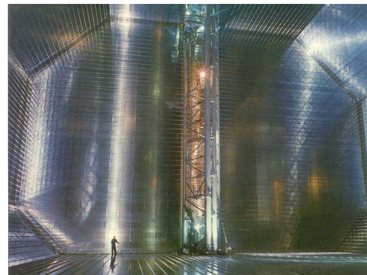
Intérieur d'une cuve de méthanier à membrane / Membrane Type LNG Tank Interior
