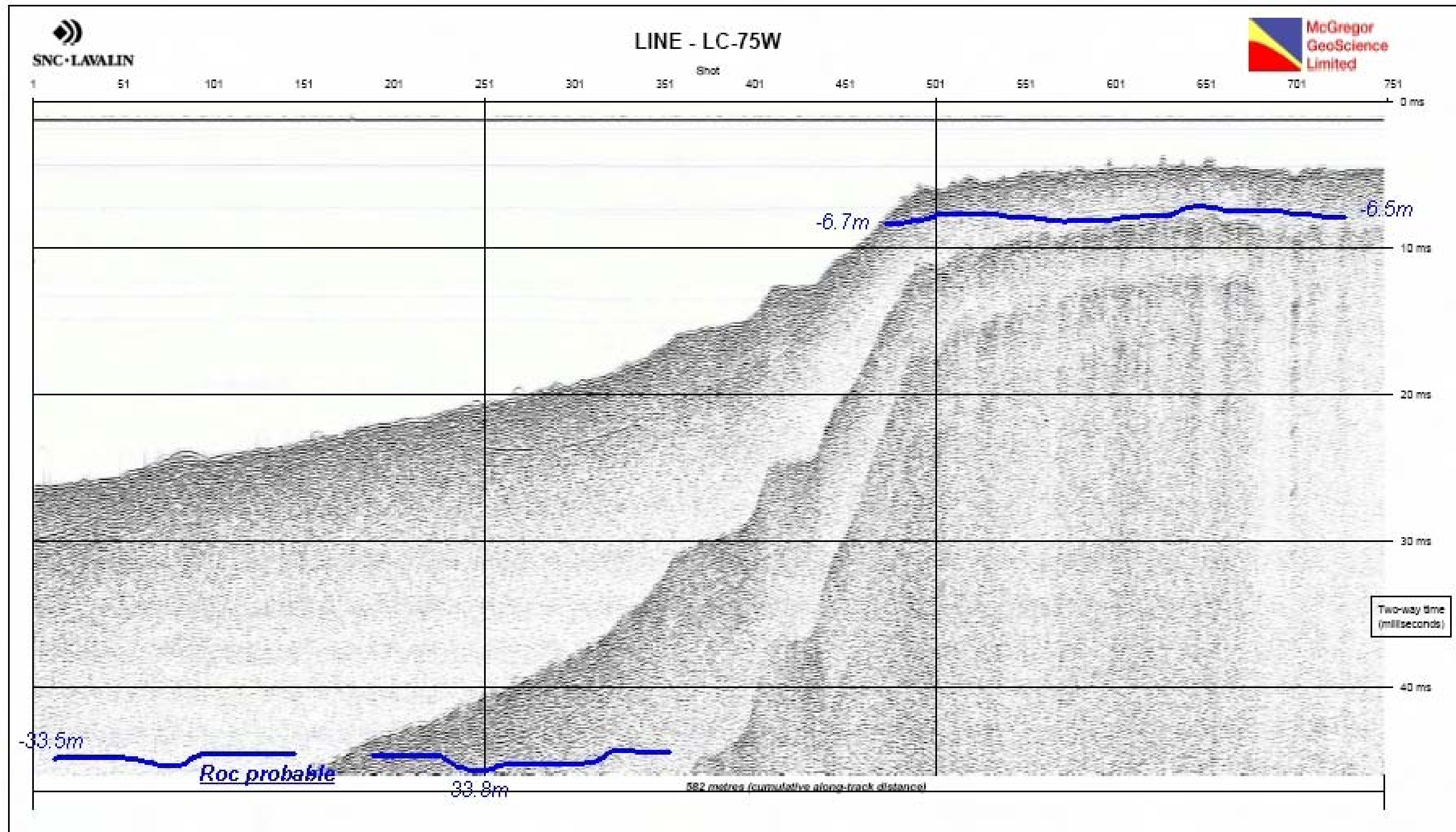
Figure 5B Interprétation des couches de matériaux observées en continu sur la ligne centrale LC-75W
