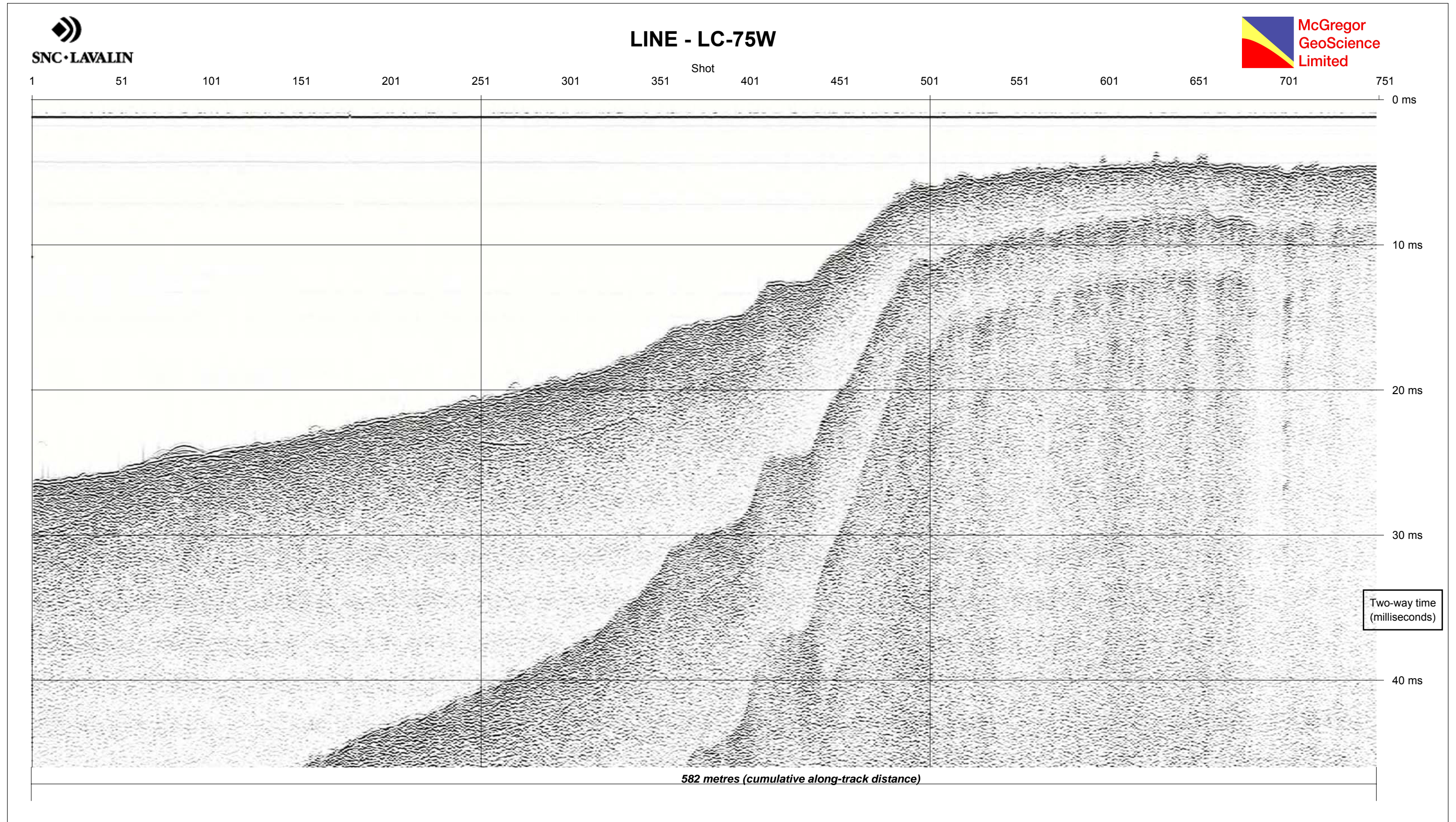
Figure 5A•Couches de matériaux observées en continu sur la ligne centrale LC-75W
