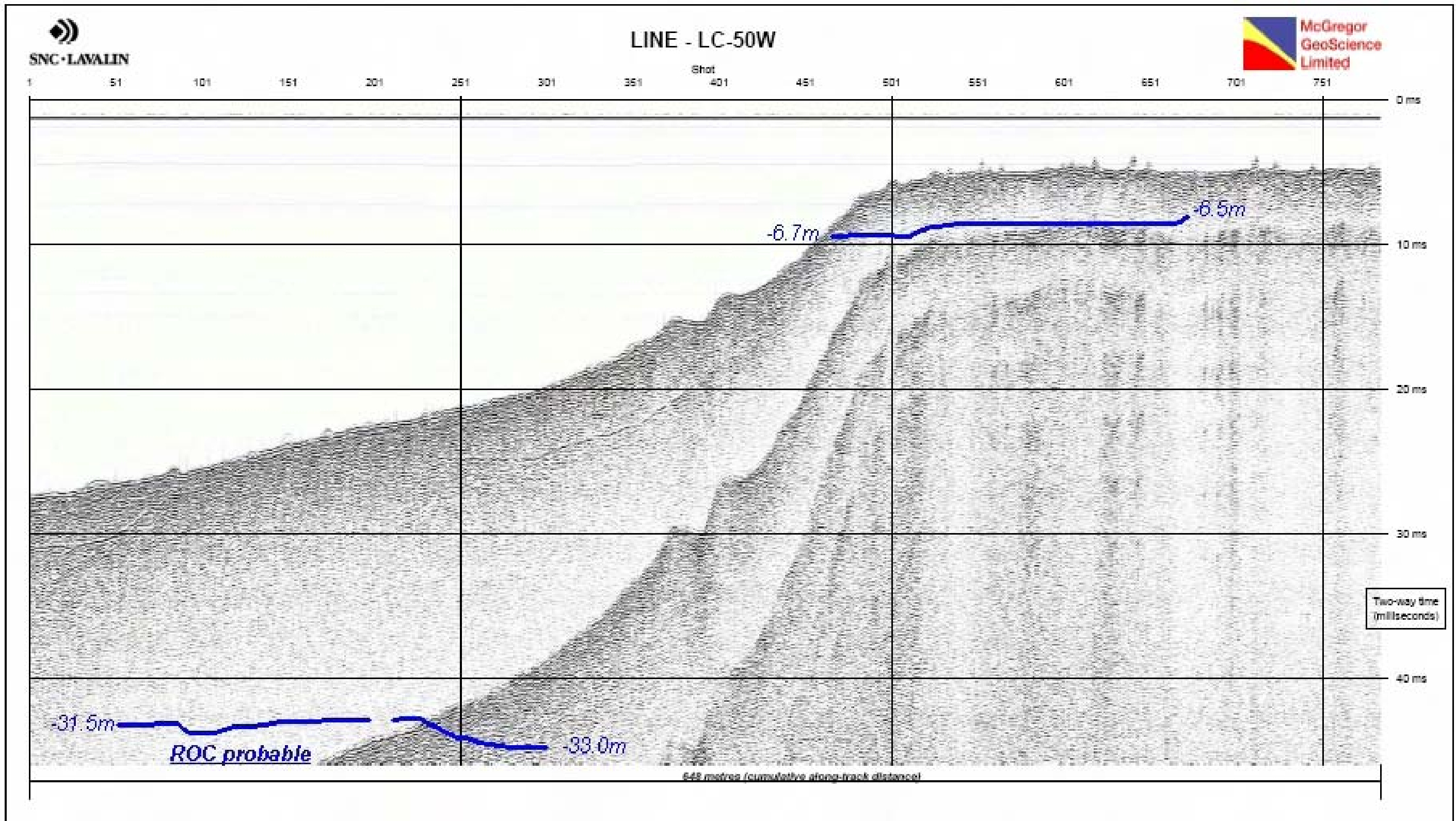
Figure 4B Interprétation des couches de matériaux observées en continu sur la ligne centrale LC-50W
