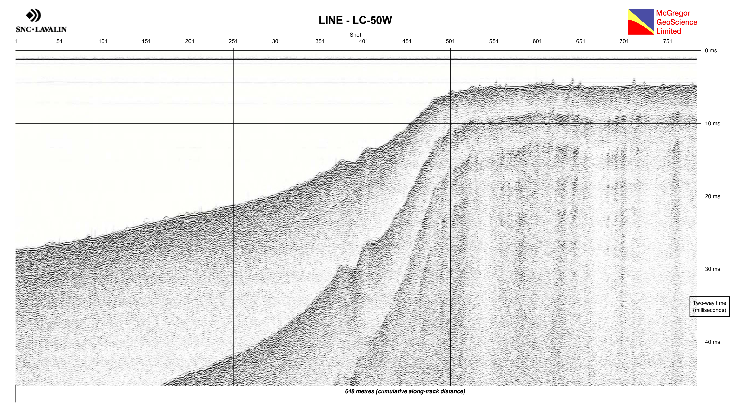
Figure 4A•Couches de matériaux observées en continu sur la ligne centrale LC-50W
