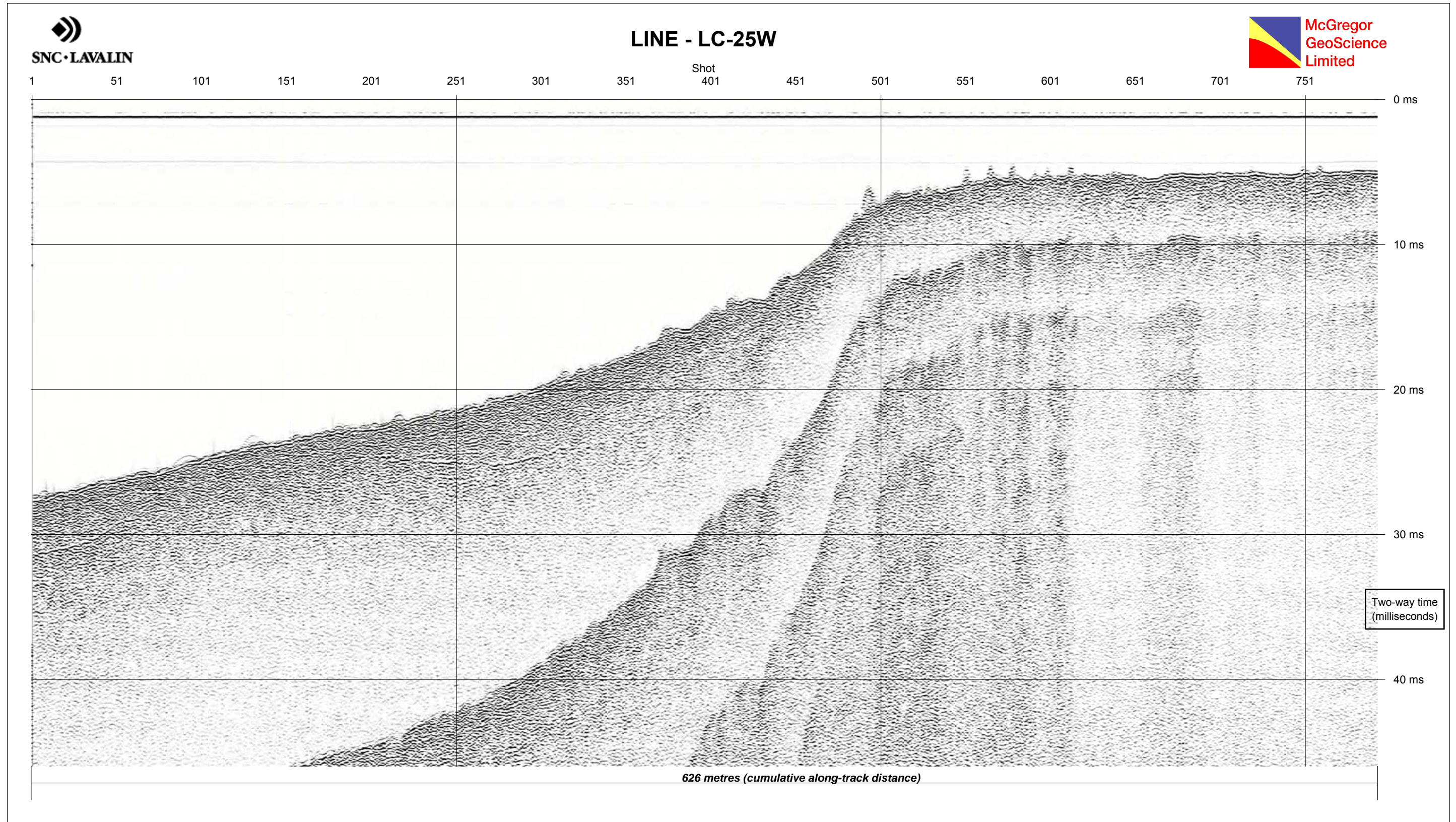
Figure 3A • Couches de matériaux observées en continu sur la ligne centrale LC-25W
