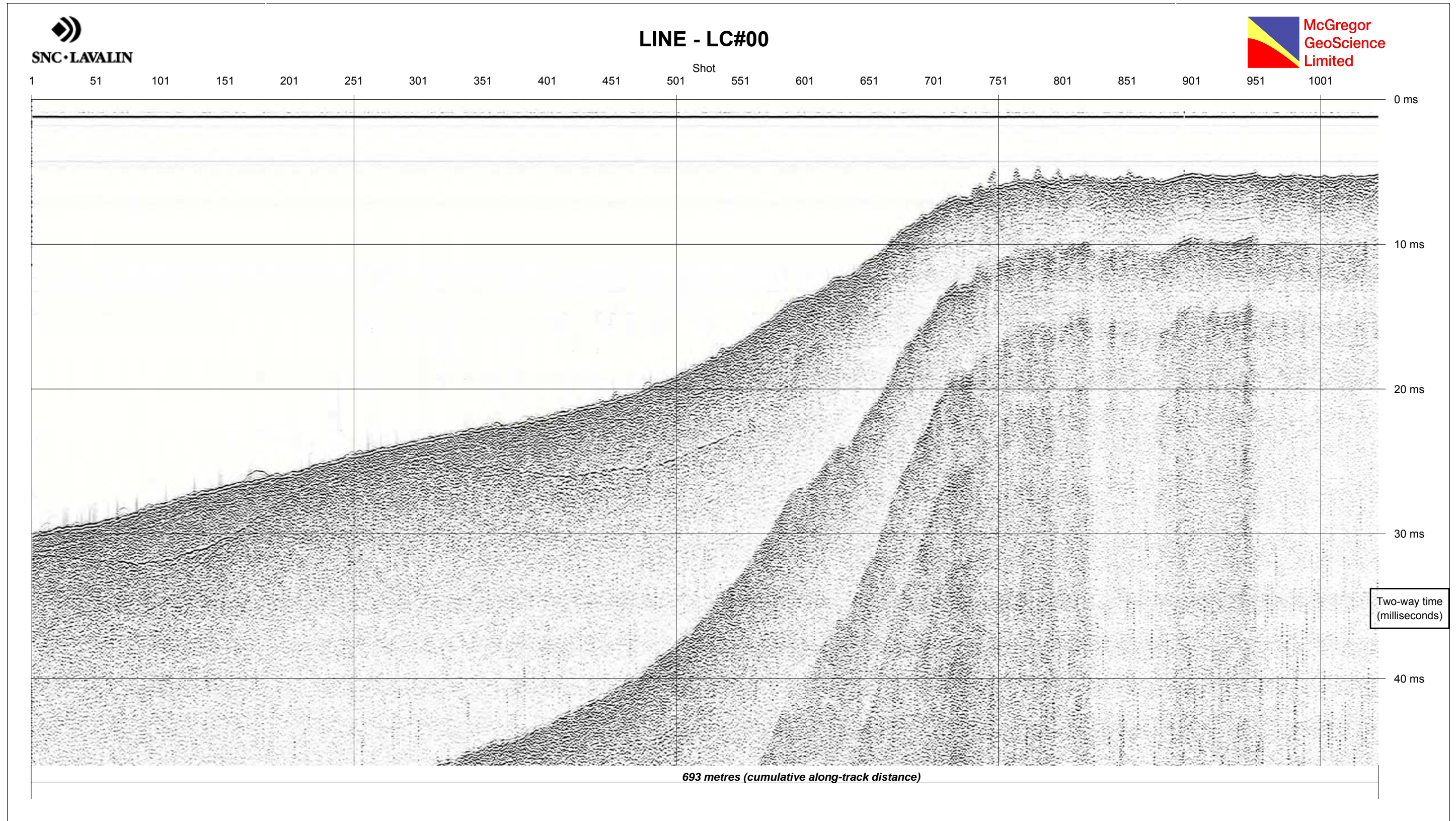
Figure 2A • Couches de matériaux observées en continu sur la ligne centrale LC+00
