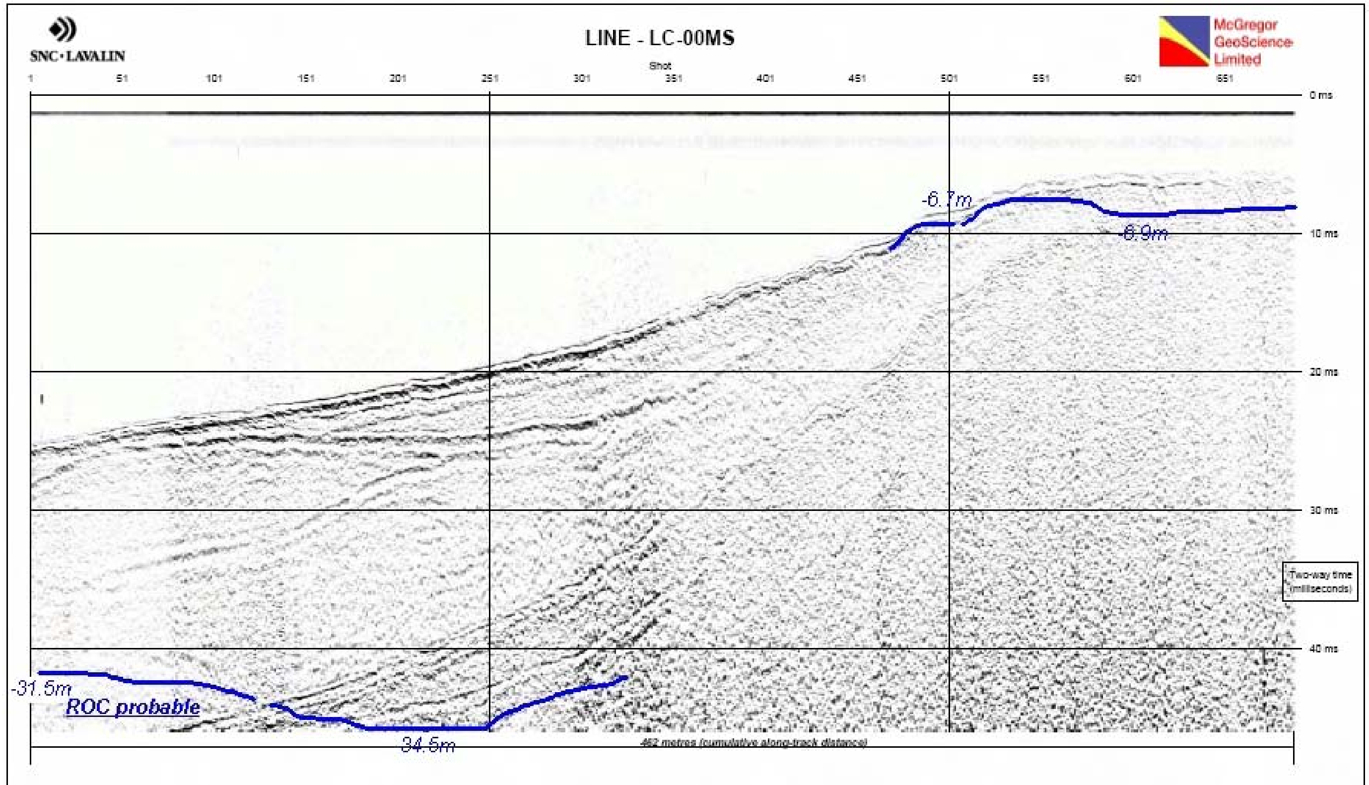
Figure 1B Interprétation des couches de matériaux observées en continu sur la ligne centrale LC+00MS
