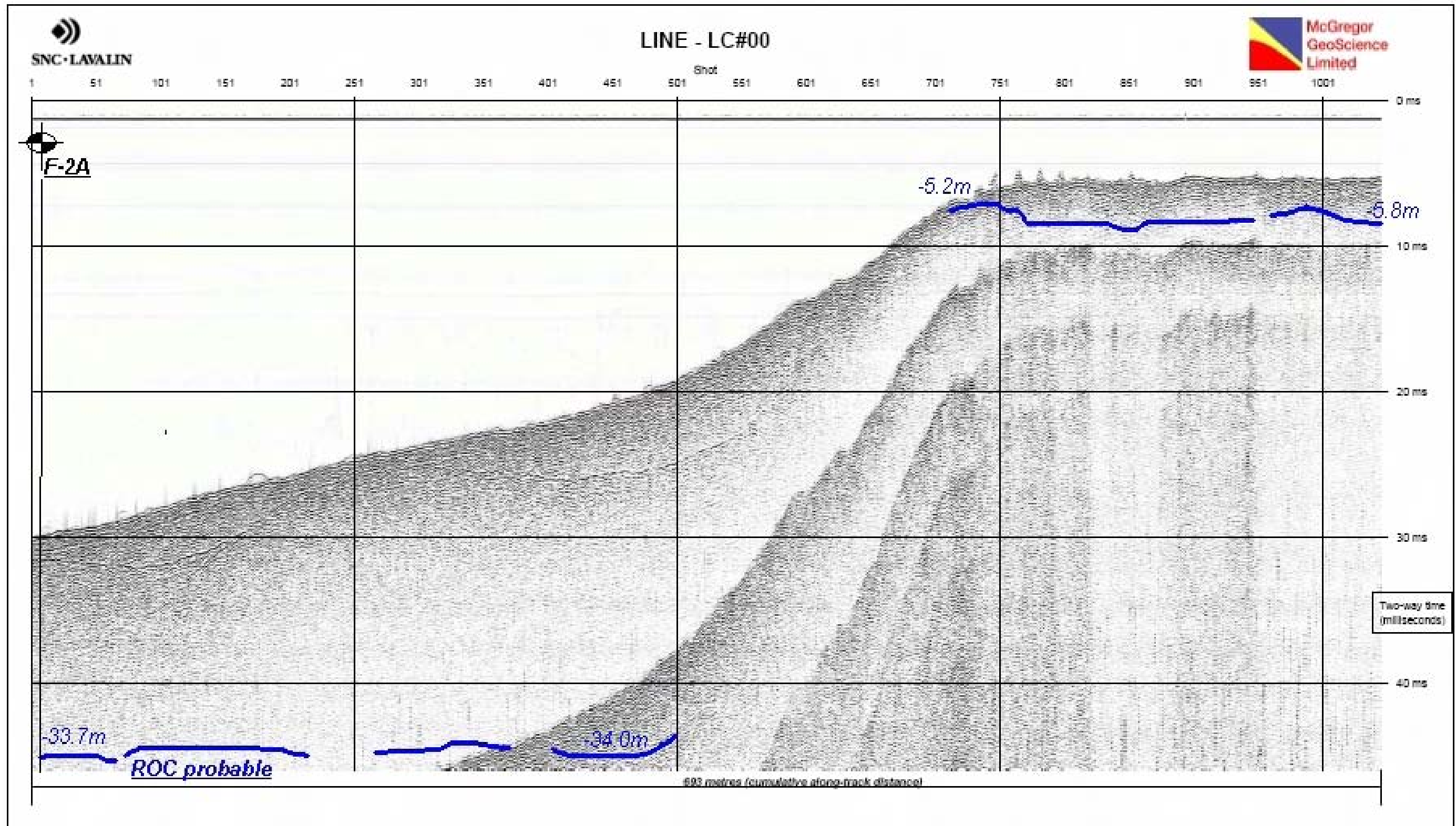
Figure 2B Interprétation des couches de matériaux observées en continu sur la ligne centrale LC+00
