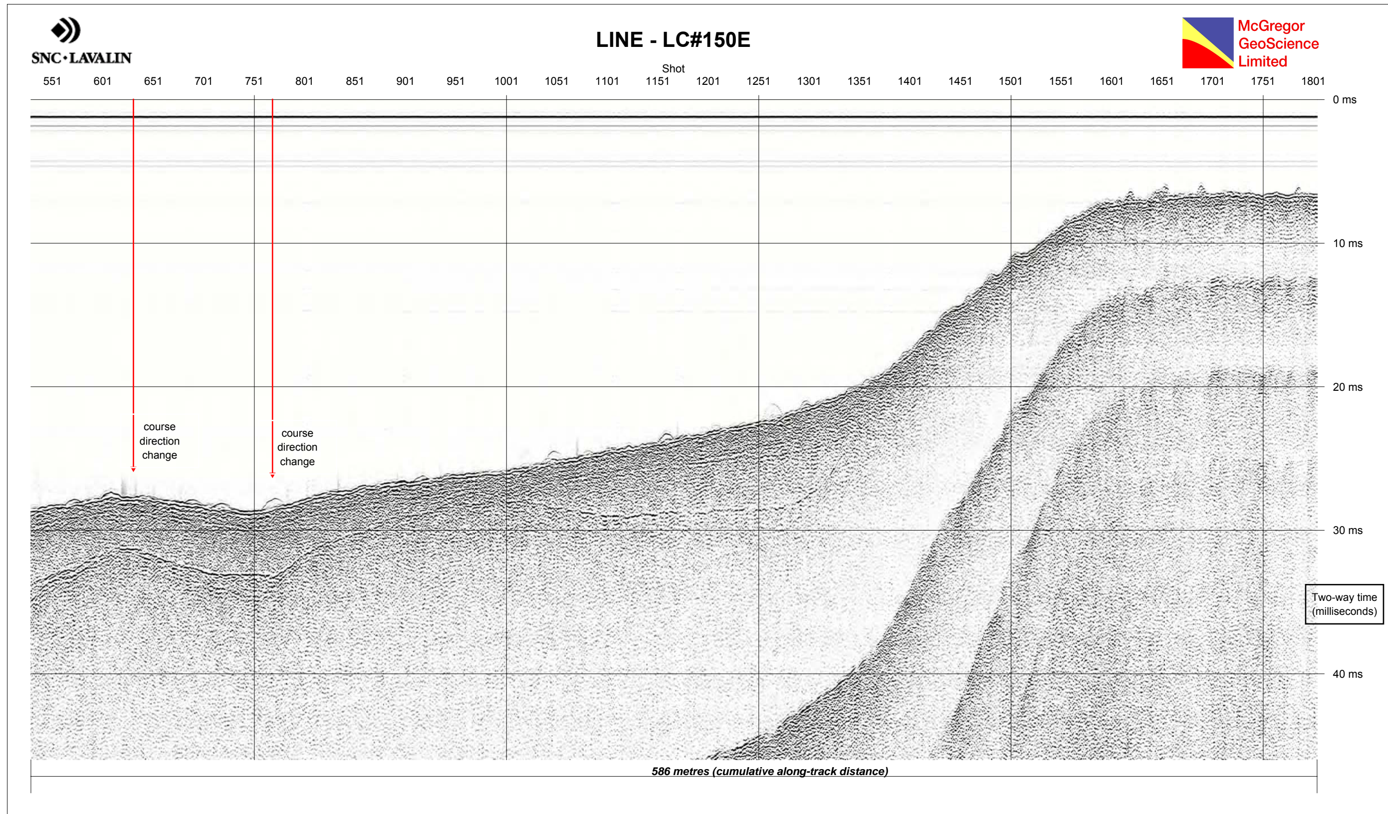
Figure 12A • Couches de matériaux observées en continu sur la ligne centrale LC-150E
