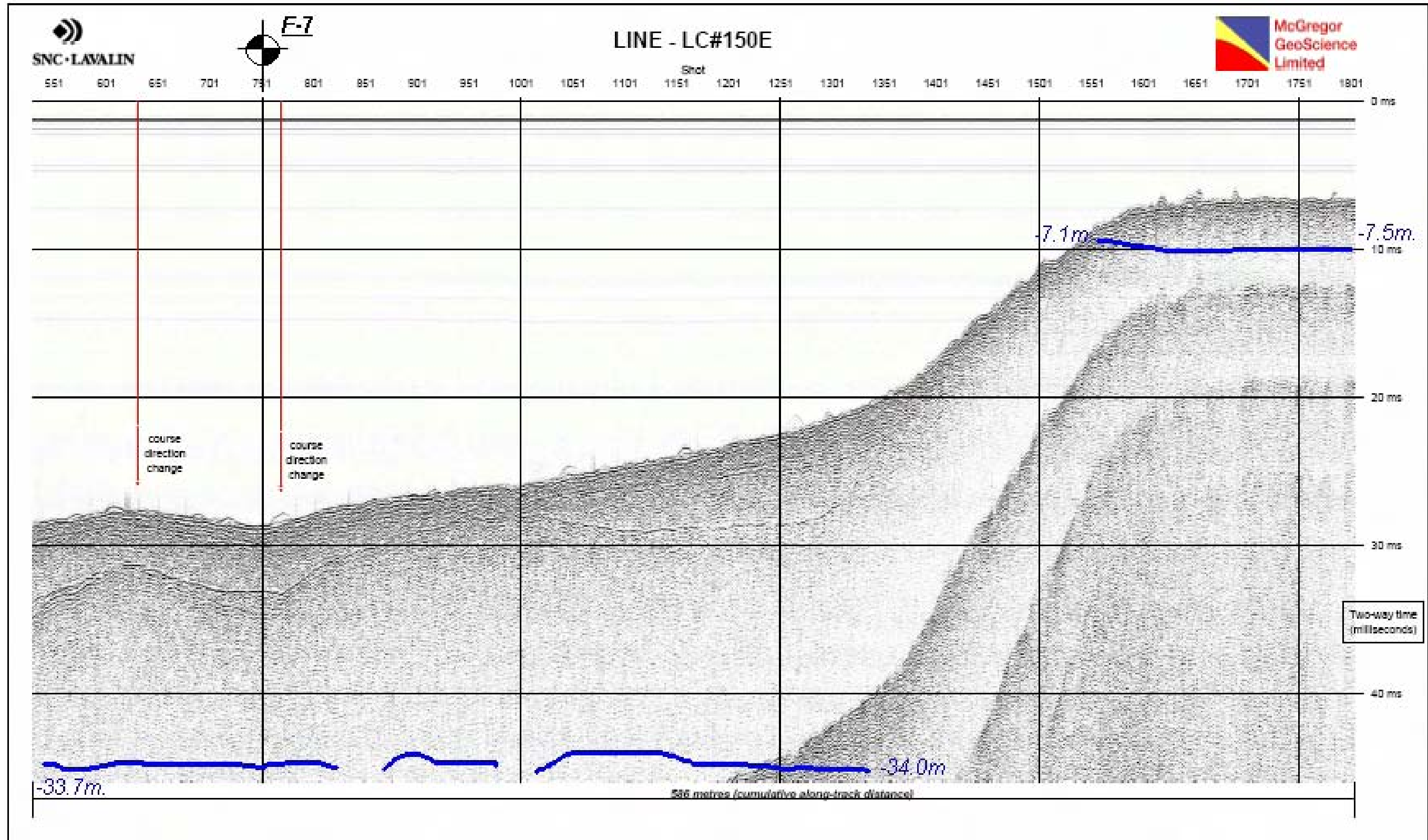
Figure 12B Interprétation des couches de matériaux observées en continu sur la ligne centrale LC-150E
