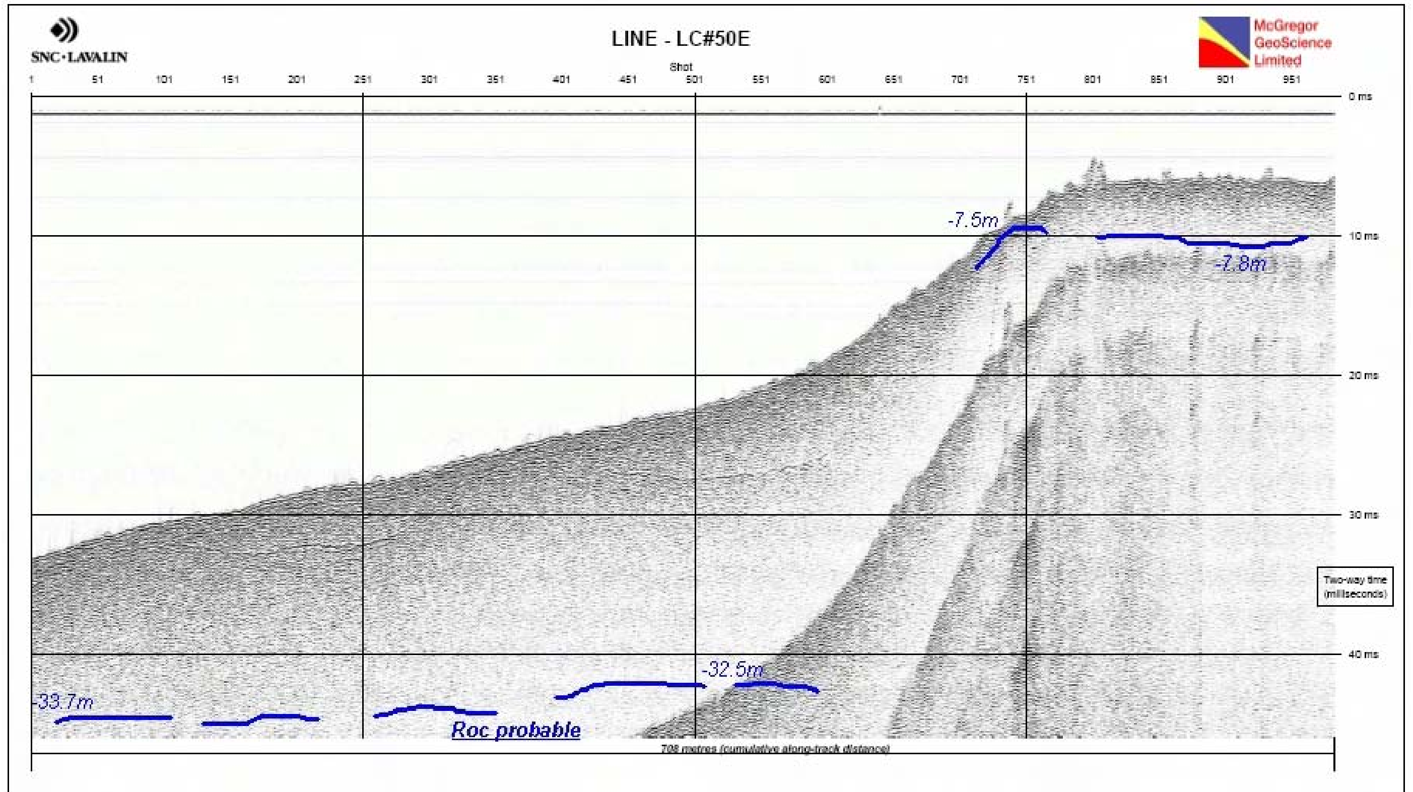
Figure 8B Interprétation des couches de matériaux observées en continu sur la ligne centrale LC-50E
