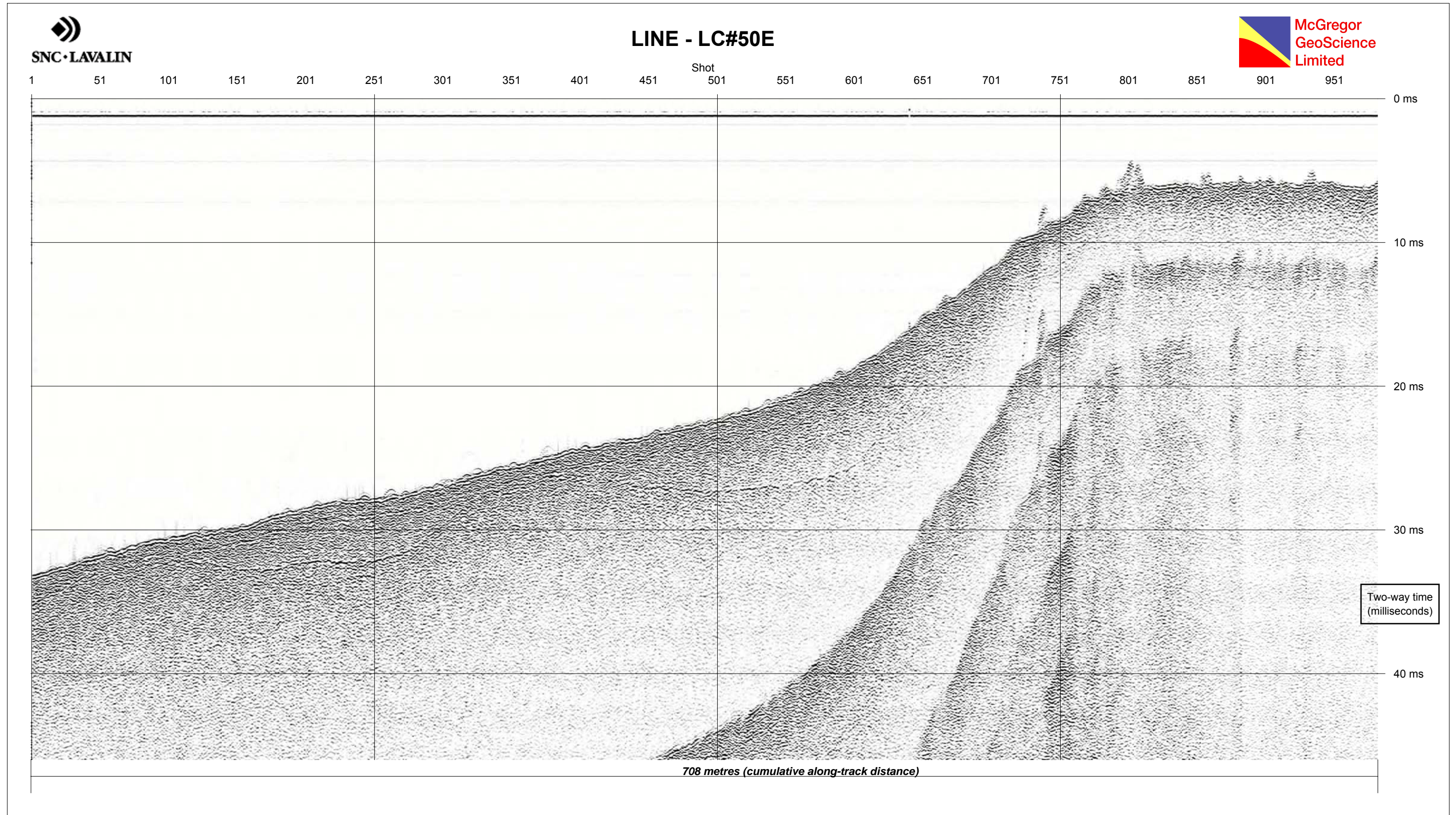
Figure 8A•Couches de matériaux observées en continu sur la ligne centrale LC-50E
