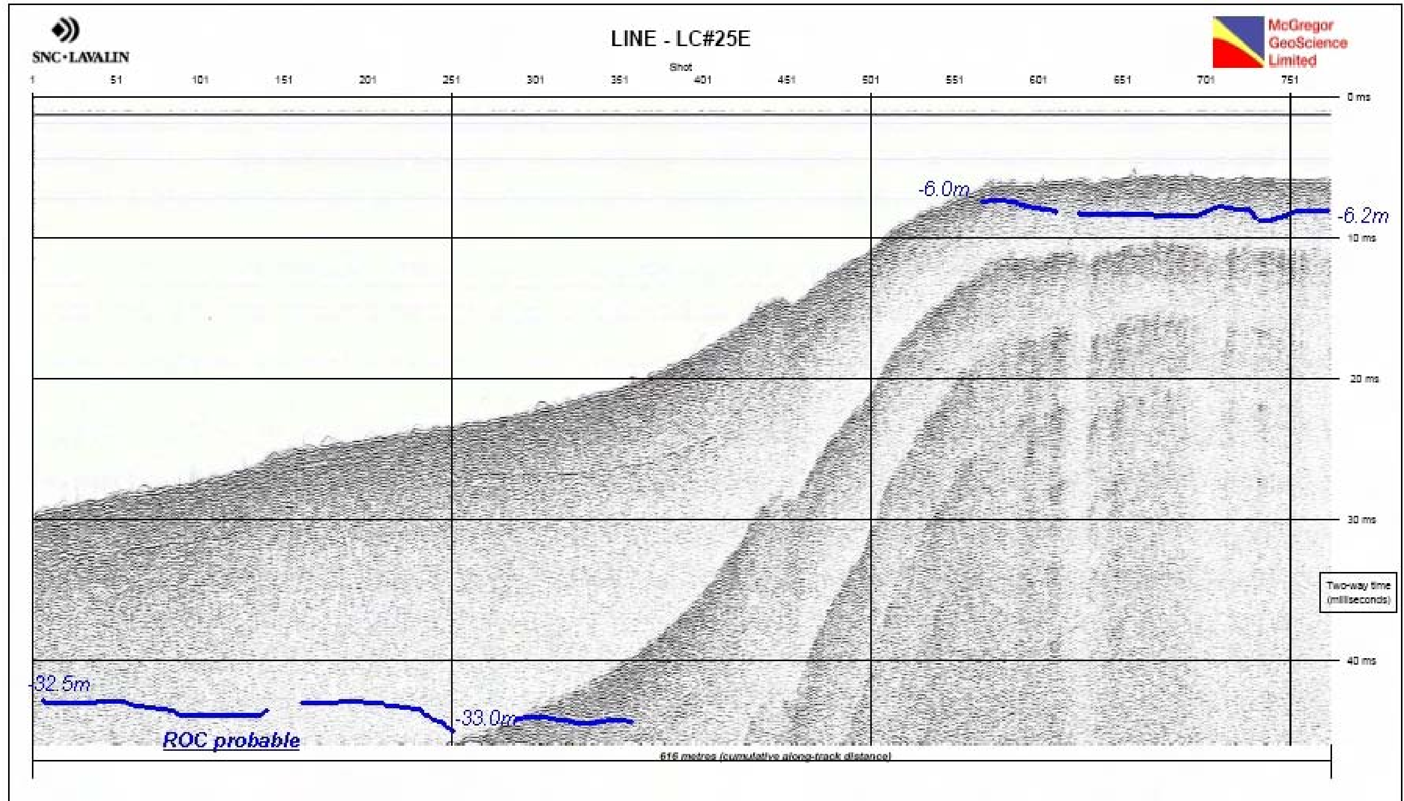
Figure 7B Interprétation des couches de matériaux observées en continu sur la ligne centrale LC-25 E
