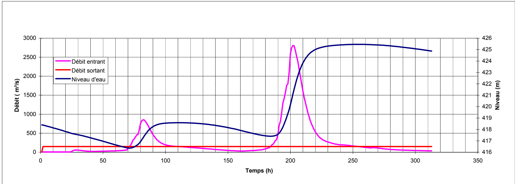
FIGURE 5.1 Hydrogramme de CMP d'été-automne dans le réservoir Pikauba Laminage Statique -Sans rupture
