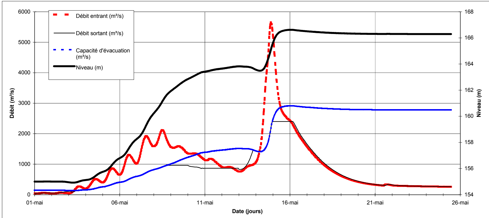
Figure 5.4 Hydrogramme de CMP de printemps dans le lac Kénogami Laminage statique - Sans rupture
