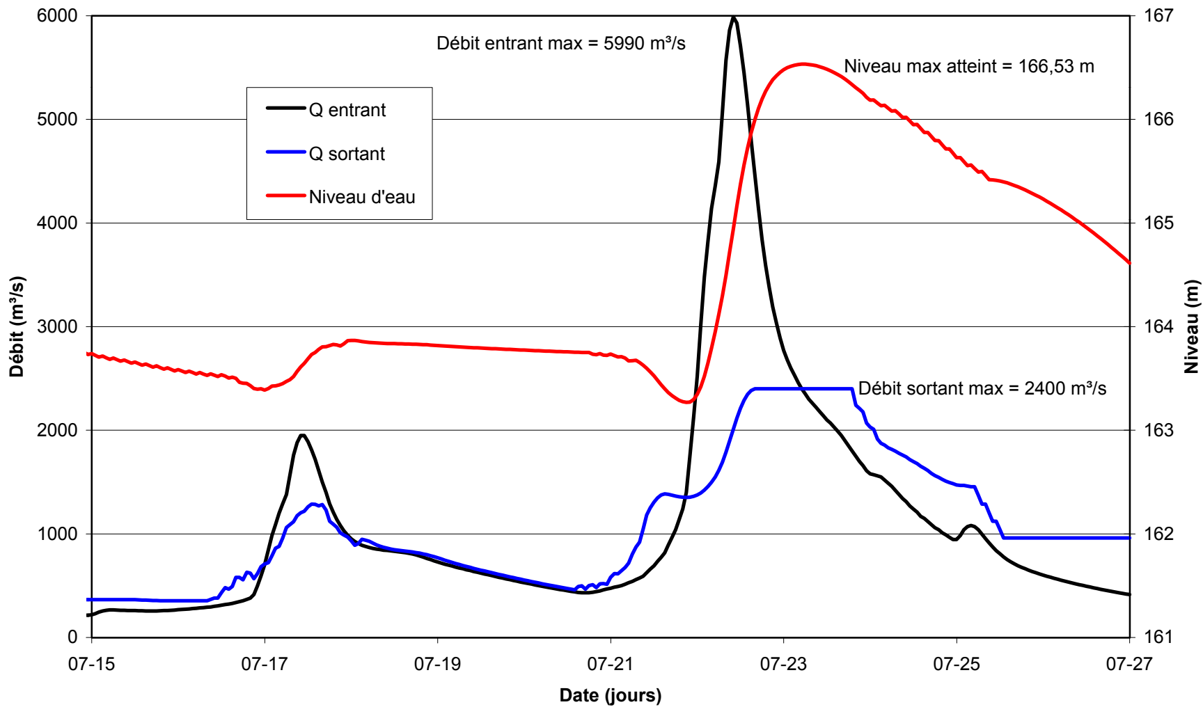
Figure 5.3 Hydrogramme de CMP d'été-automne dans le lac Kénogami Laminage statique - Sans rupture
