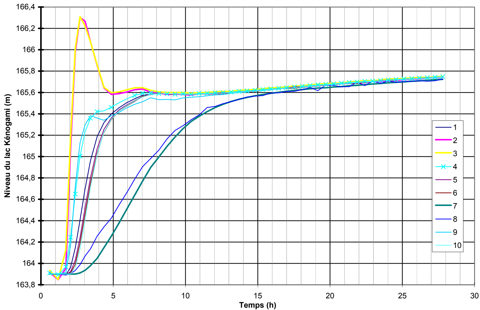
Figure 5.6 Rupture en temps sec du barrage Pikauba Simulation hydrodynamique du niveau d'eau dans le lac Kénogami à l'aide du modèle Serum
