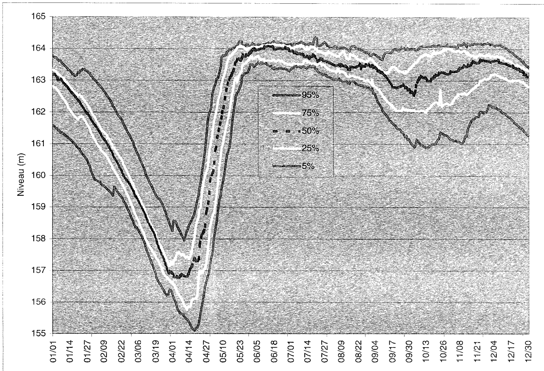
Pourcentage de non-dépassement des niveaux au lac Kénogami (station 061001 au barrage Portage-des-Roches) de 1983 à 2002
