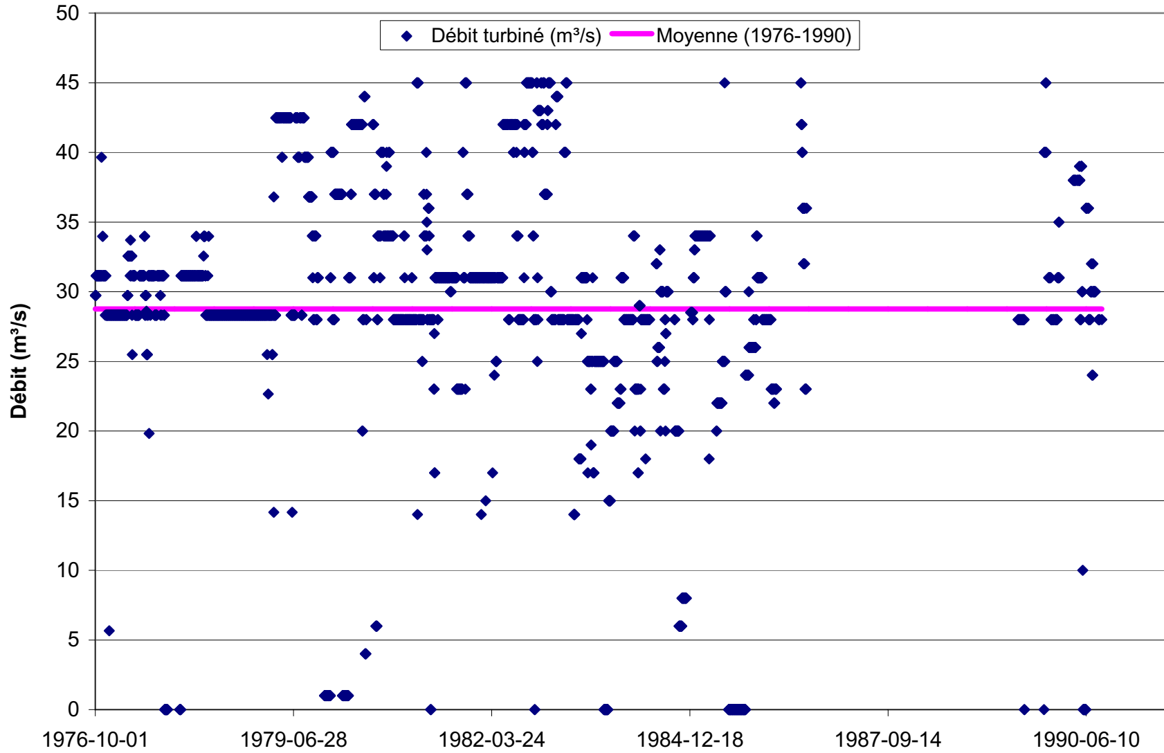
Débits turbinés journaliers à Pont Arnaud (m 3 /s)
