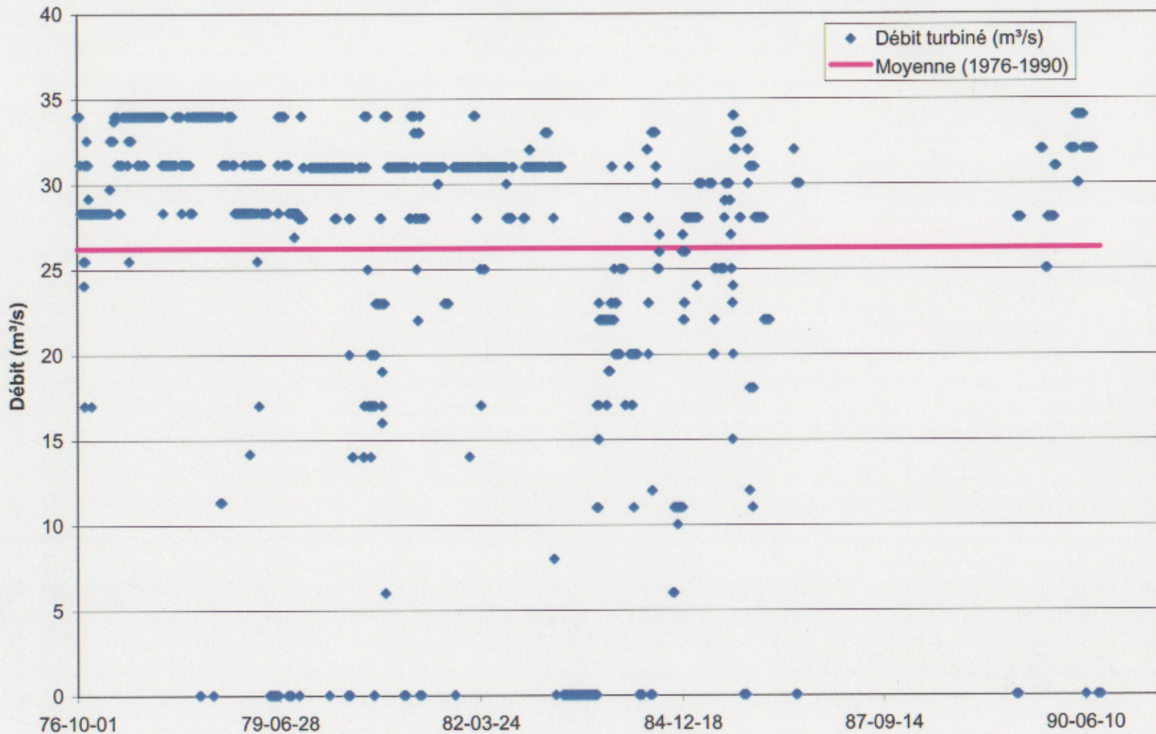
Débits turbinés journaliers à Chute Garneau ( \text{m}^3/\text{s} )
