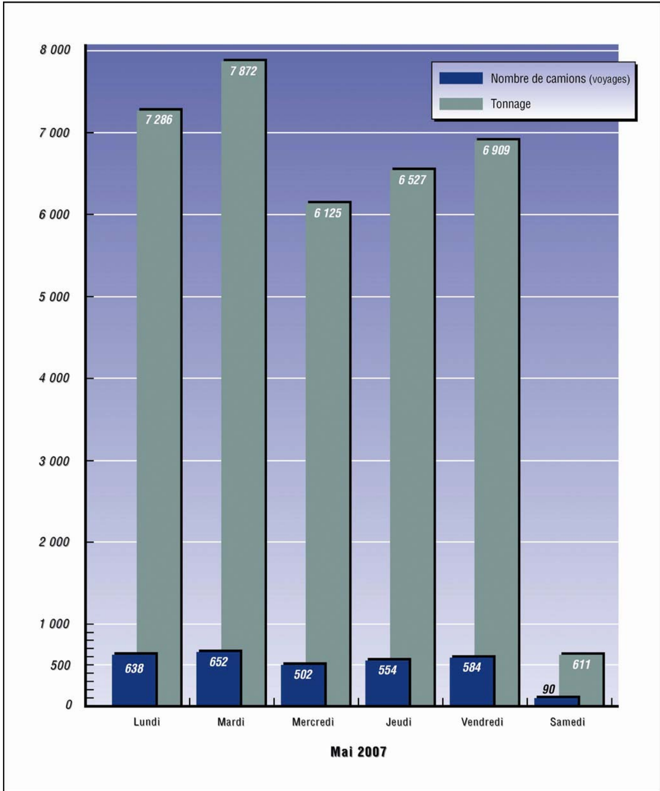
Figure 3.8 : Nombre moyen de camions et tonnages enregistrés au LET de BFI, pour une semaine de mai 2007
