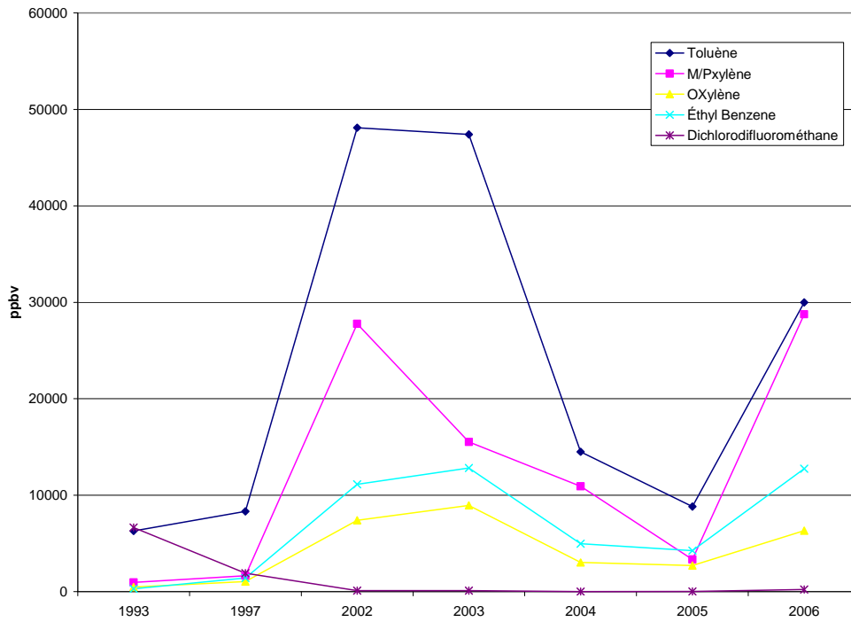
Figure 3 : Variation des concentrations de toluène, M/P xylène, oxylène, éthyl benzène et dichlorodifluorométhane dans le biogaz échantillonné à BFI-UTL
