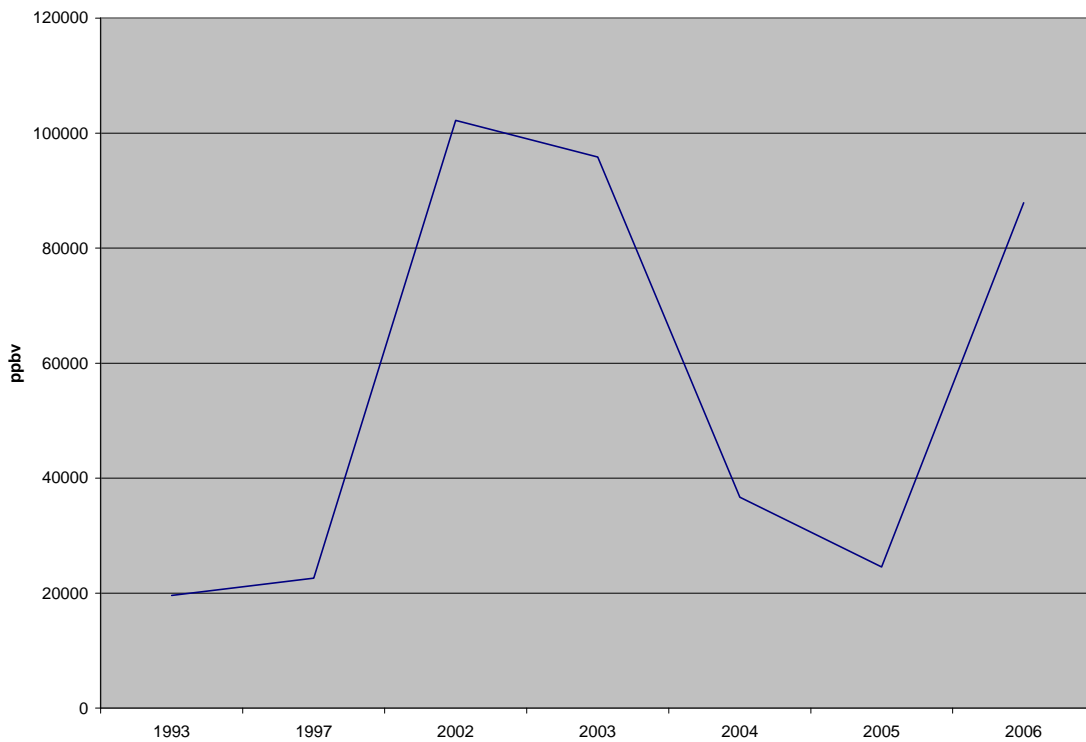
Figure 2 : Variation de concentration des COV (Méthode TO-14a) dans le biogaz échantillonné à BFI-UTL
