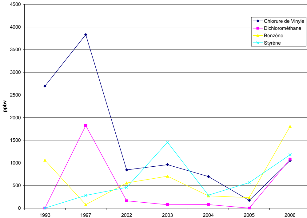
Figure 4 : Variation des concentrations chlorure de vinyle, dichlorométhane, benzène et styrène dans le biogaz échantillonné au site d'enfouissement à BFI-UTL
