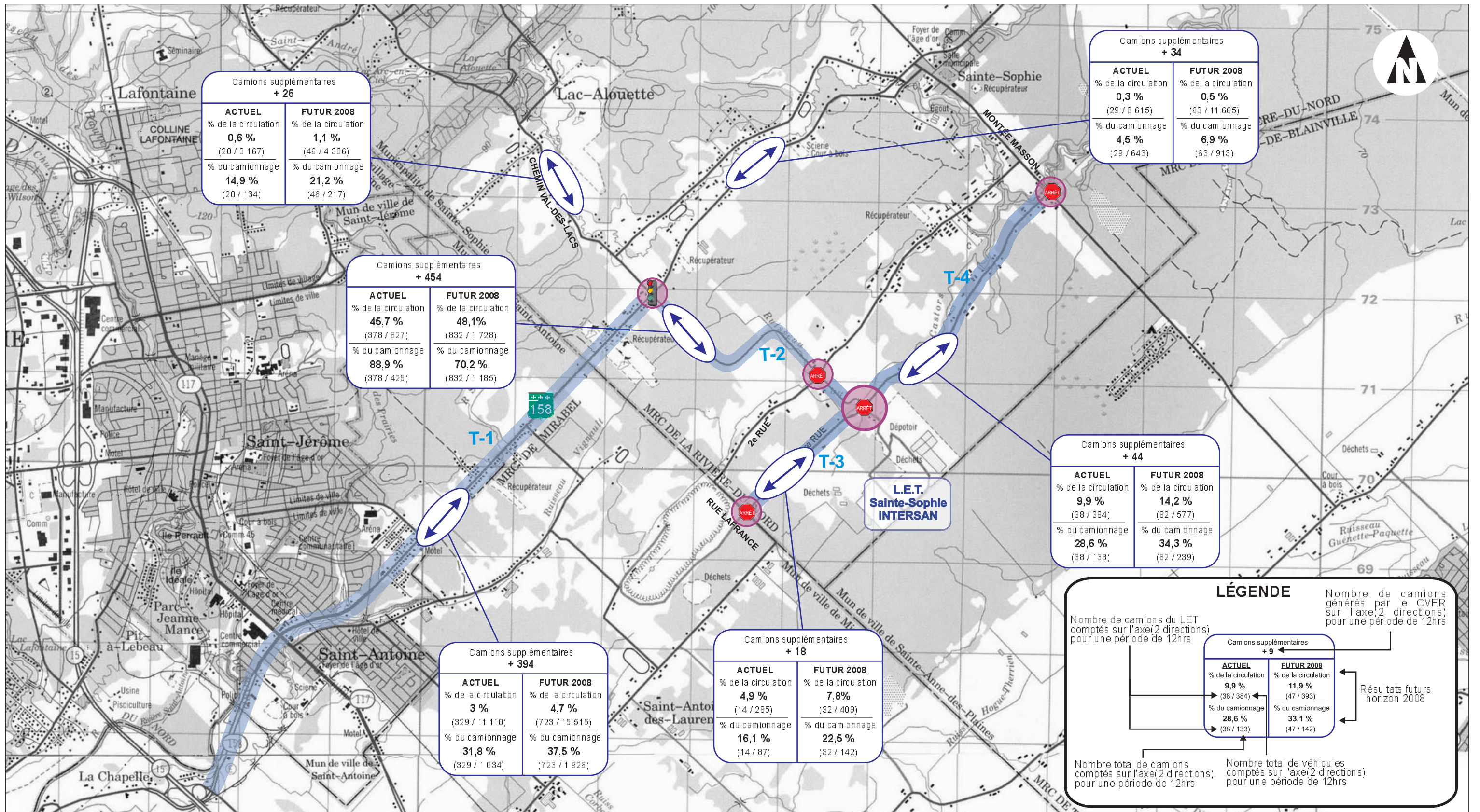
IMPACT DU CVER SUR LES DÉBITS JOURNALIERS Achalandage en période de construction - jour de semaine Horizon 2008
