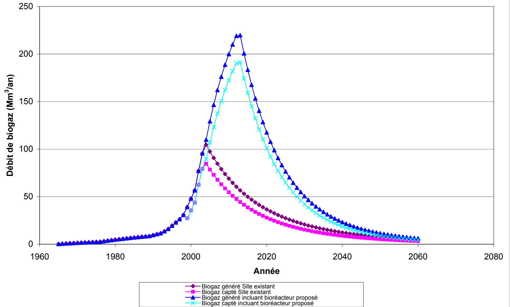
Figure 2-3: Courbe de génération et de captage du biogaz - Bioréacteur proposé - CVER de Sainte-Sophie
