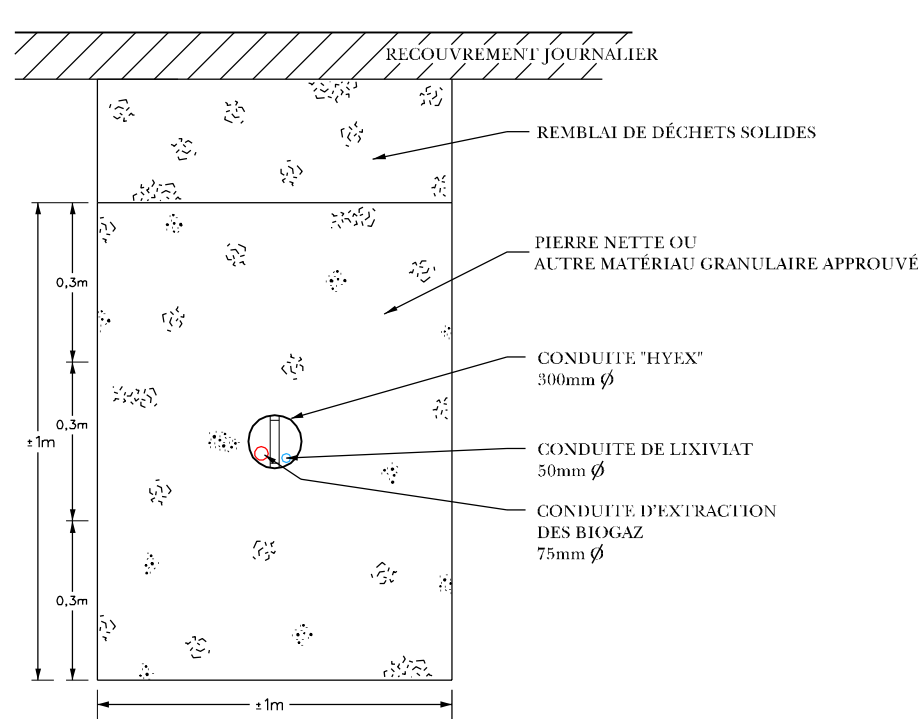
CONDUITE "HYEX" COUPE TYPE DE TRANCHEE AUCUNE ÉCHELLE
