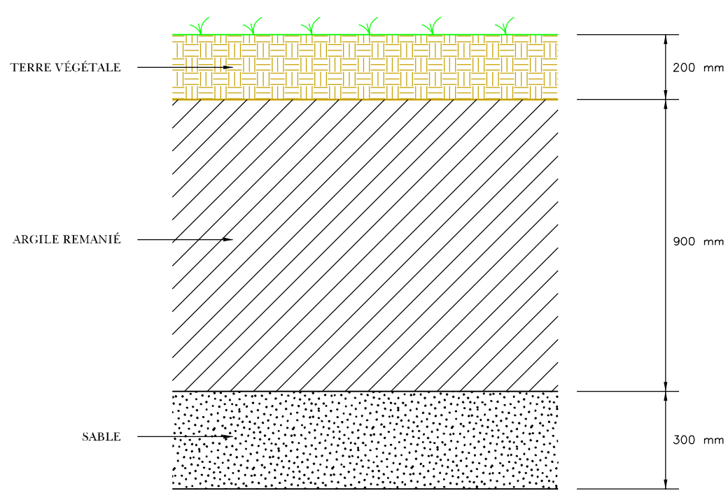
COUPE TYPE RECROUVREMENT FINAL AUCUNE ÉCHELLE
