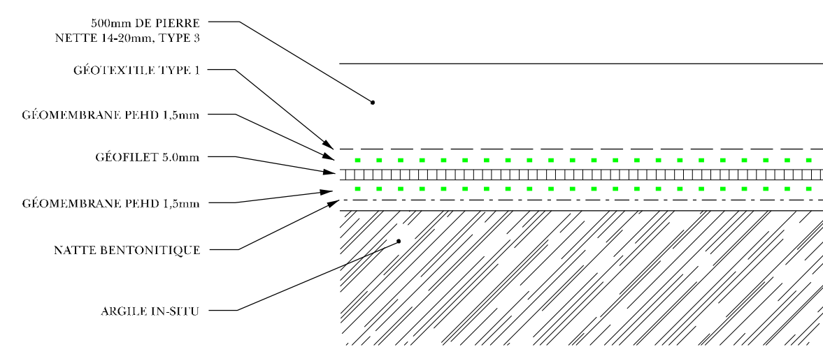
COUPE TYPE DU SYSTÈME D'IMPERMÉABILISATION AUCUNE ÉCHELLE
