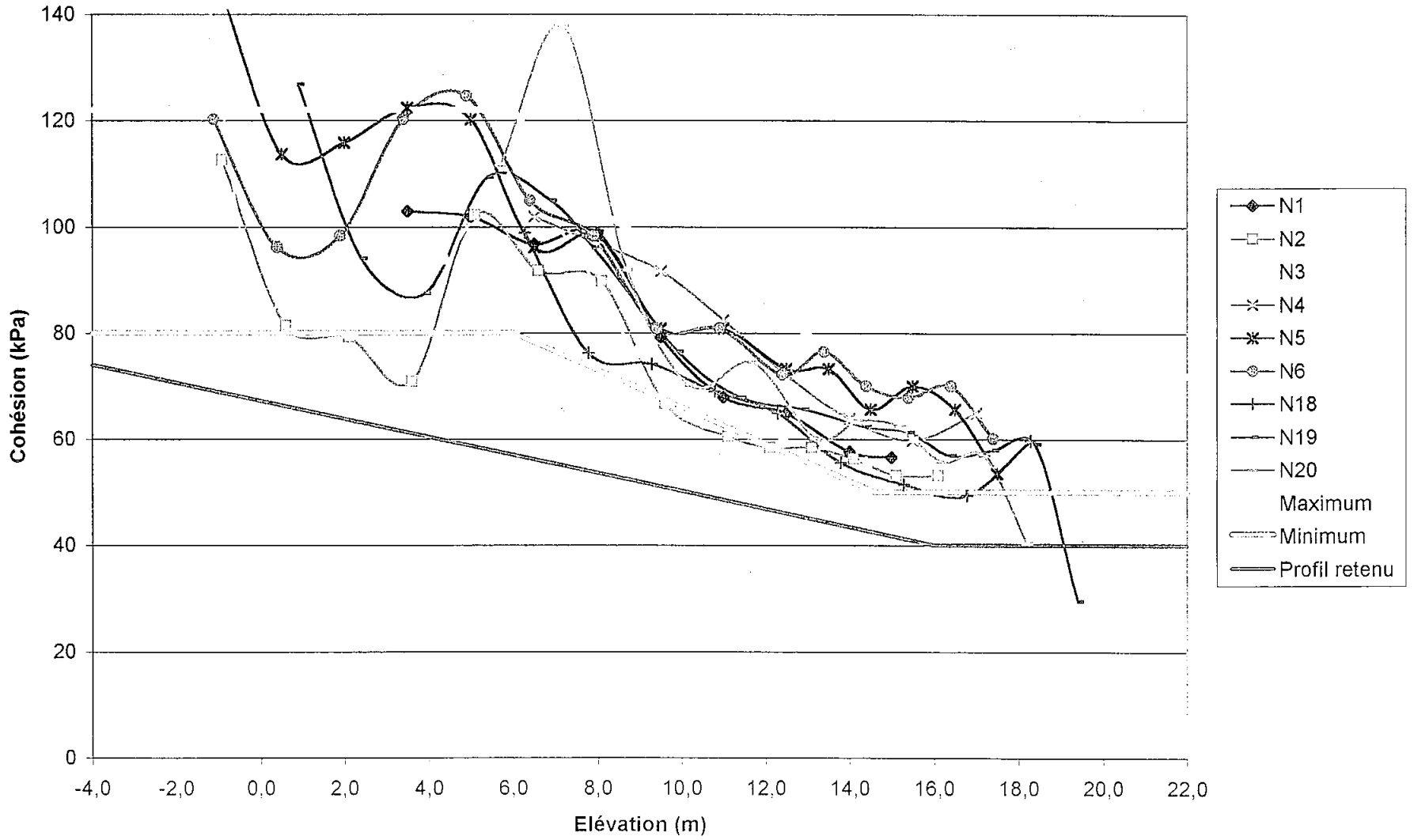
Figure 7-1-Essais Nilcon -Extérieur Ouest
