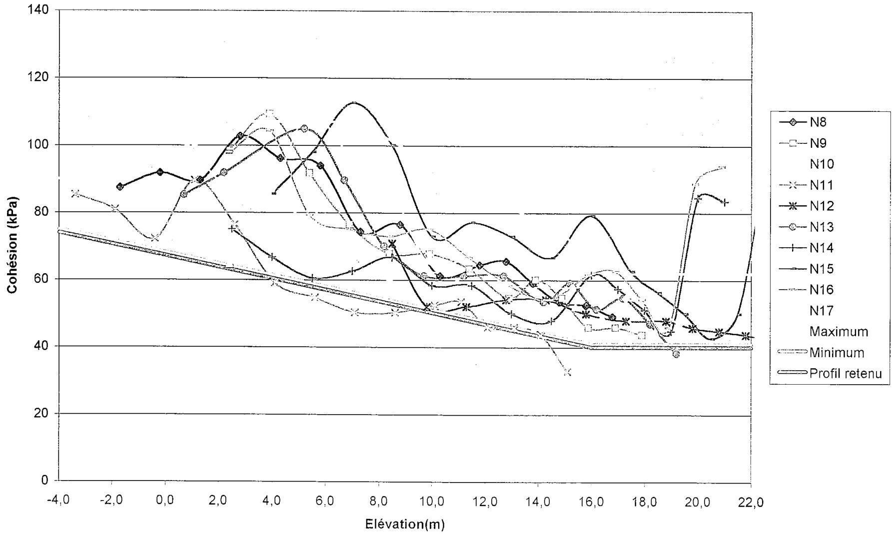
Figure 7-2-Essais Nilcon-Extérieur Est
