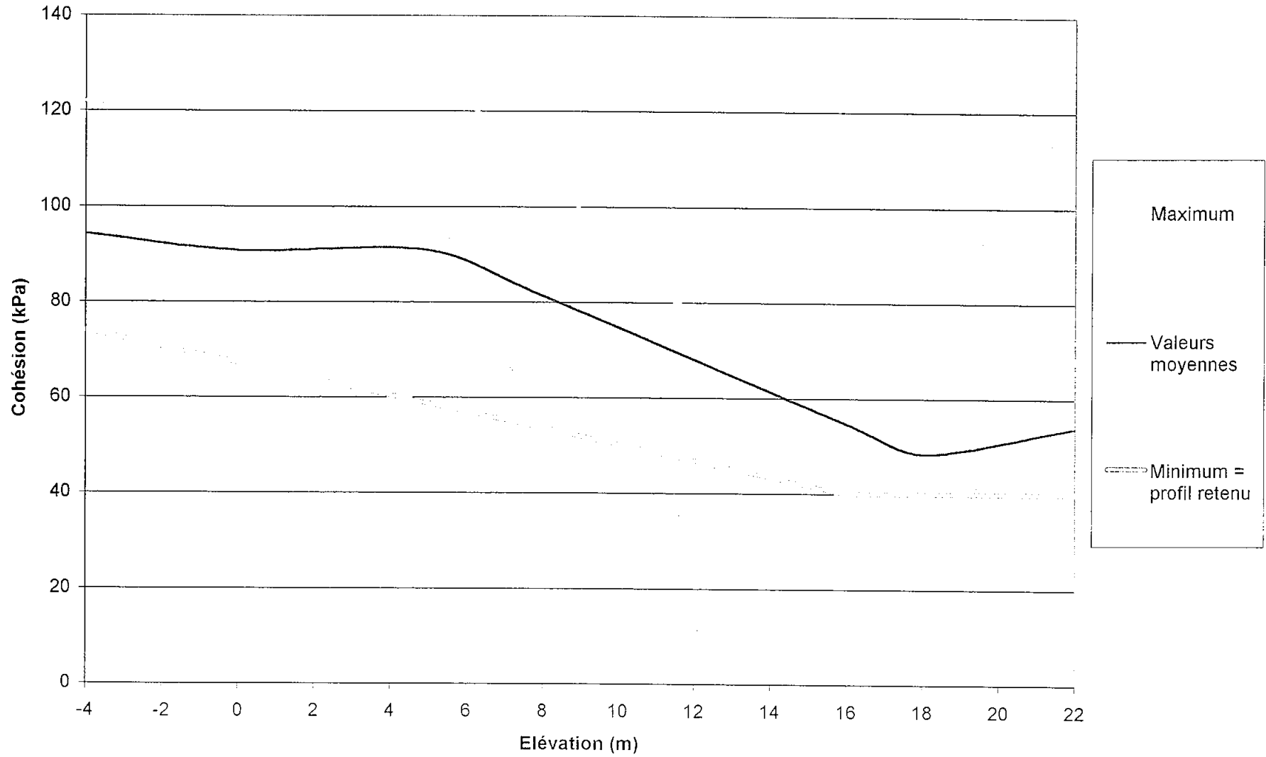
Figure 7-5-Essais Nilcon - Récapitulatif
