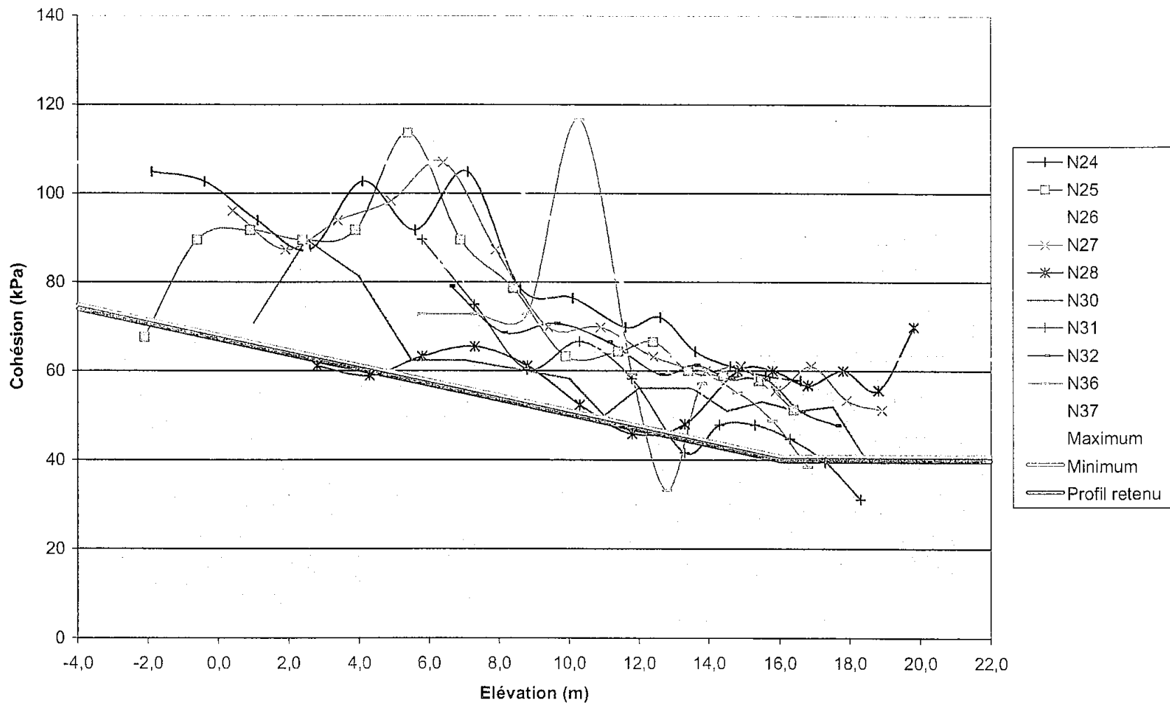
Figure 7-3-Essais Nilcon-Bande centrale
