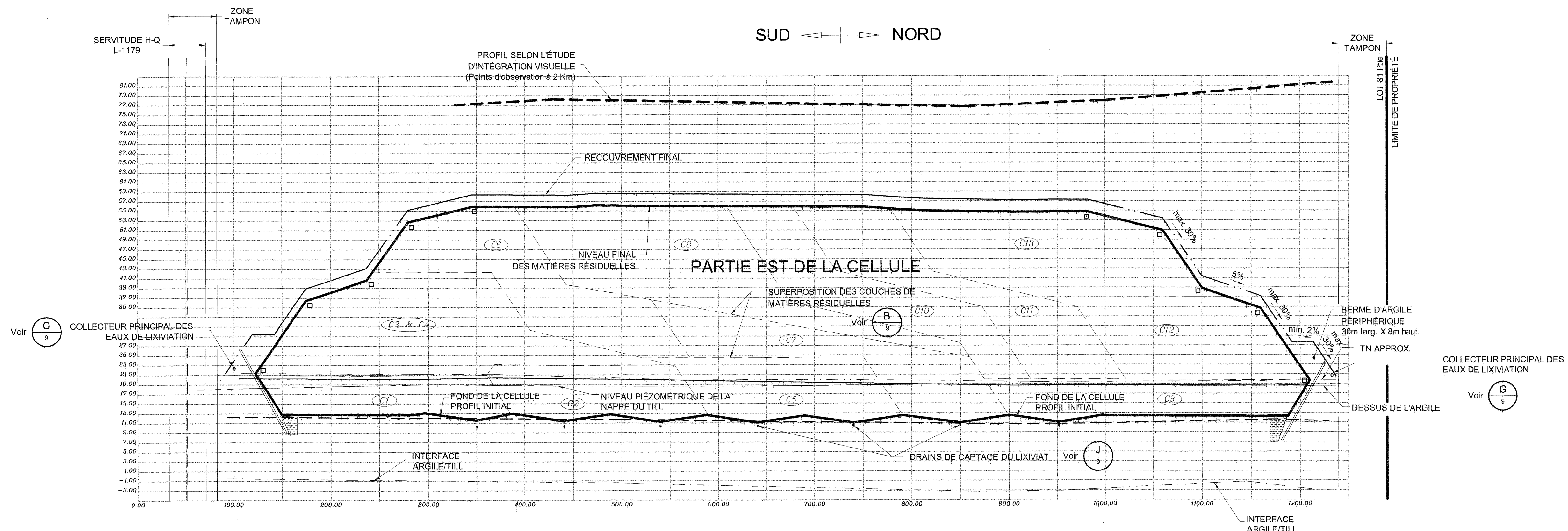
COUPE D-D AVANT TASSEMENT
