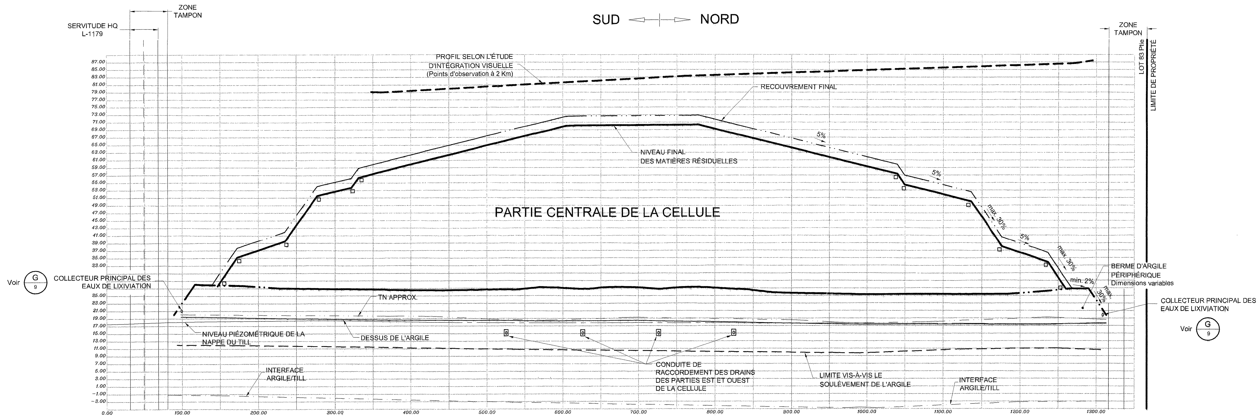
COUPE C-C AVANT TASSEMENT
