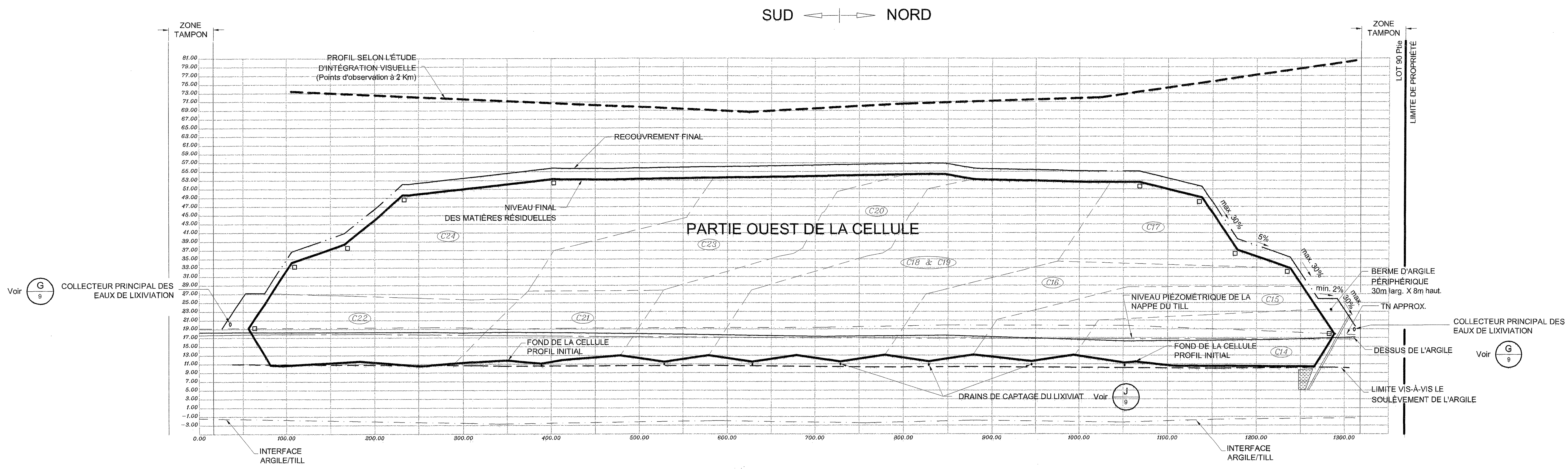
COUPE B-B AVANT TASSEMENT
