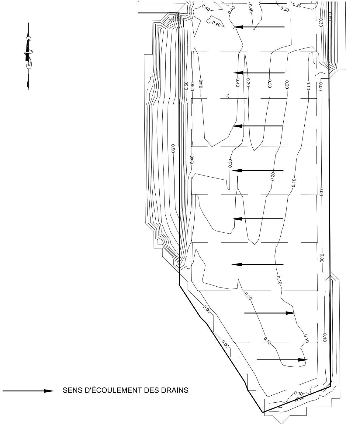
Figure 1.0 AMPLITUDE DES TASSEMENTS ABSOLUS DU FOND DE LA CELLULE APRÈS OPTIMISATION DE LA CAPACITÉ D'ENFOUISSEMENT DU SECTEUR EST
