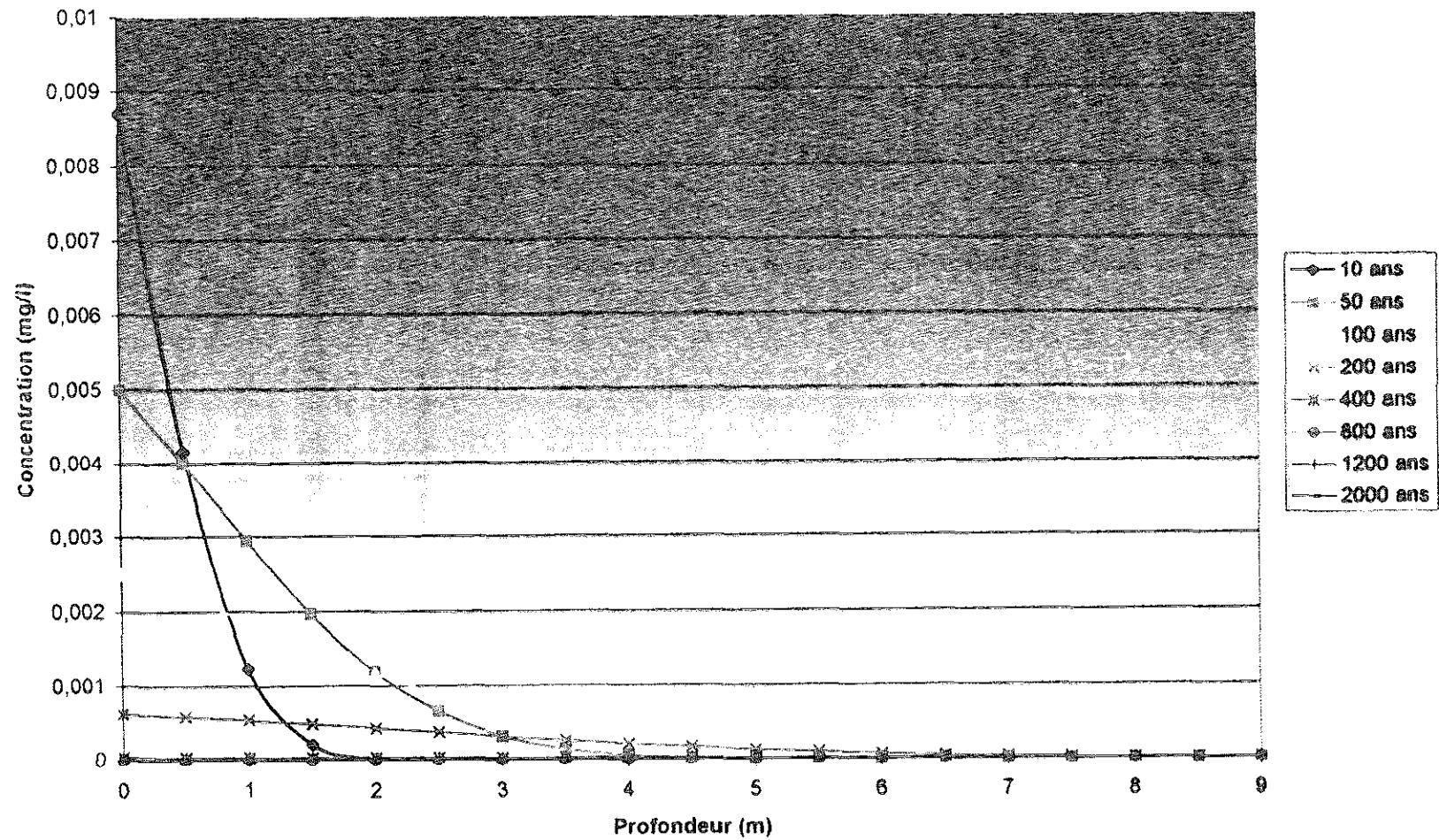
Fig 5.2 Profil des concentrations du 1,4-Dichlorobenzène en fonction du temps sous les bassins de traitement de lixiviat
