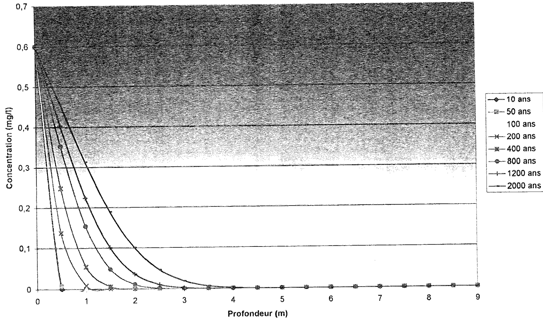
Fig 5.1 Profil des concentrations du Plomb en fonction du temps sous les bassins de traitement de lixiviat
