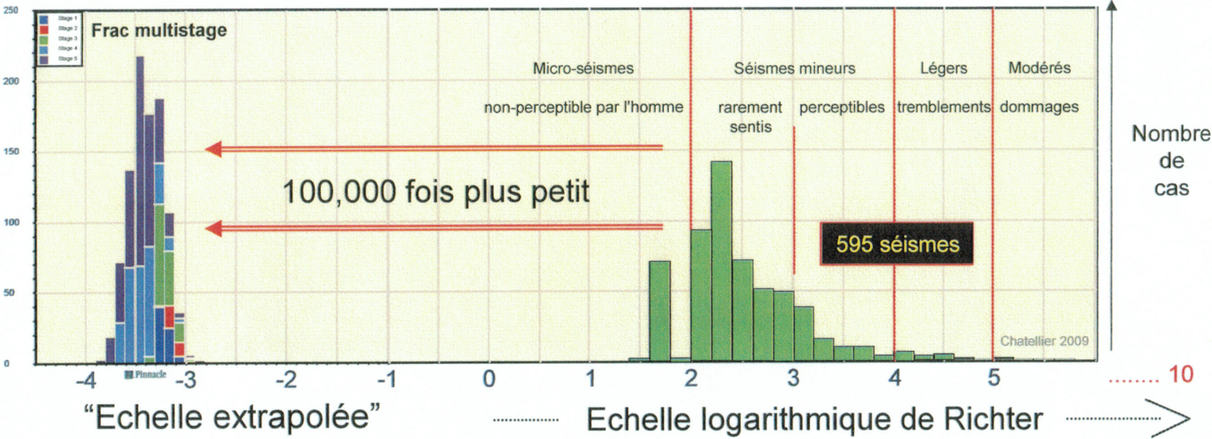
Fracturation hydraulique dans un puits à 2km de profondeur (shale gas)
