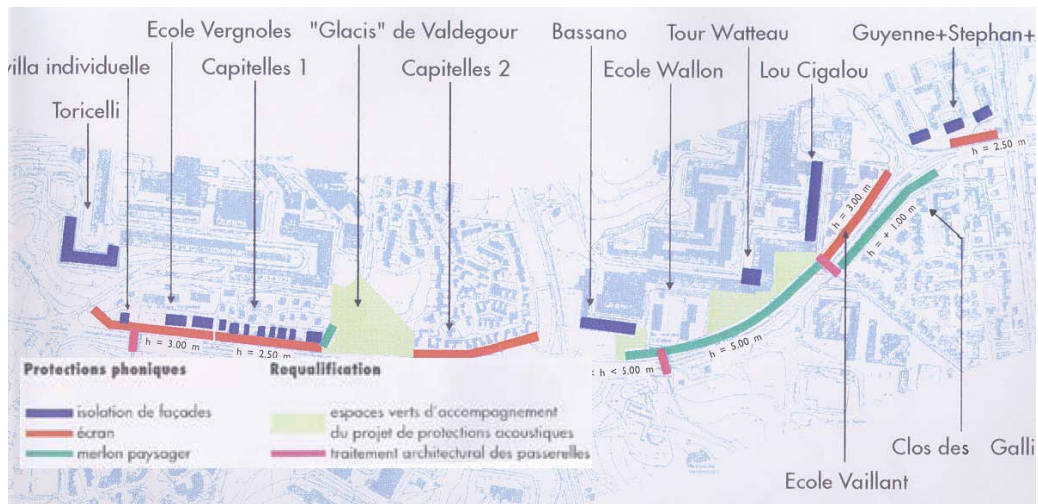
Figure 5.5 Plan conceptuel d'aménagement de la route
