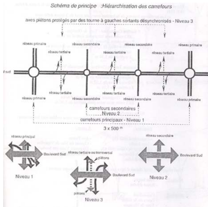
Figure 6.4 Types de carrefours et d'articulations
