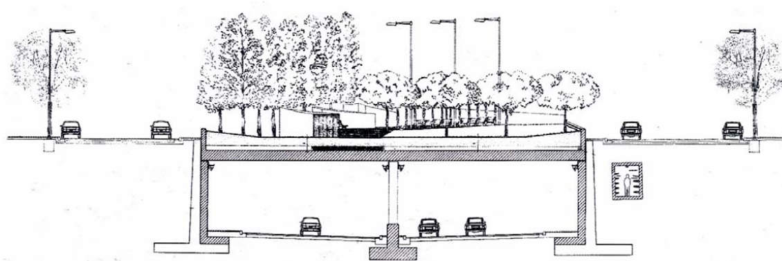
Figure 2.9 Coupe transversale de la Ronda de la montagne Source : HENRY, Guy. Barcelone : dix années d'urbanisme, la renaissance d'une ville , 1992, p. 109
