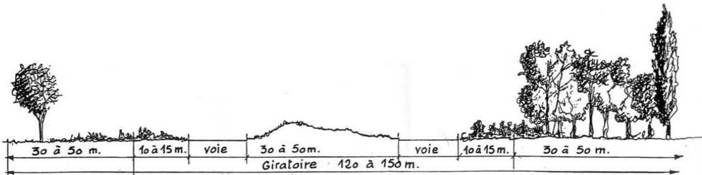
Figure 6.7 Coupe de principe d'un carrefour d'entrée d'une zone d'activités
