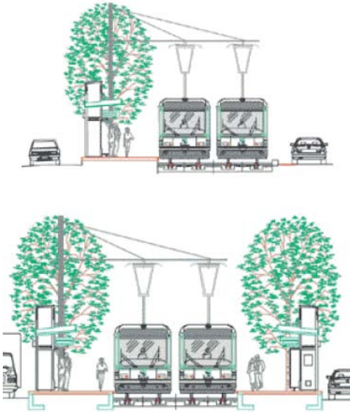
Figures 4.10 et 4.11 Présentation en coupe de deux stations (tramway en position axiale)
